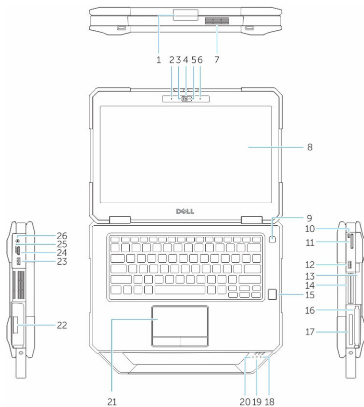
Slika 1. Pregled sustava
