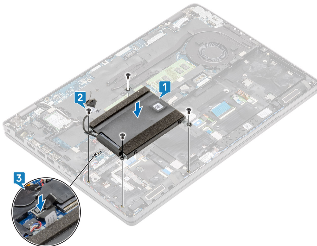
Figura4. Instalar o disco rígido
