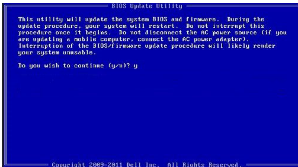
Figur 4. DOS BIOS-opdateringsskærmen
