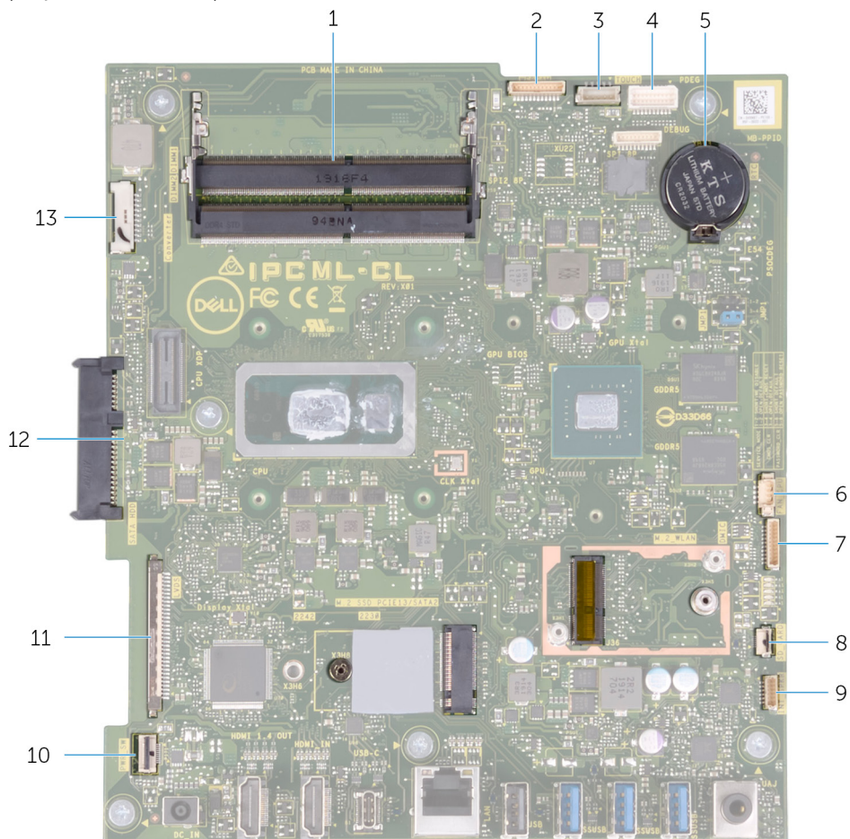
Skica 1. Priključki sistemske plošče
