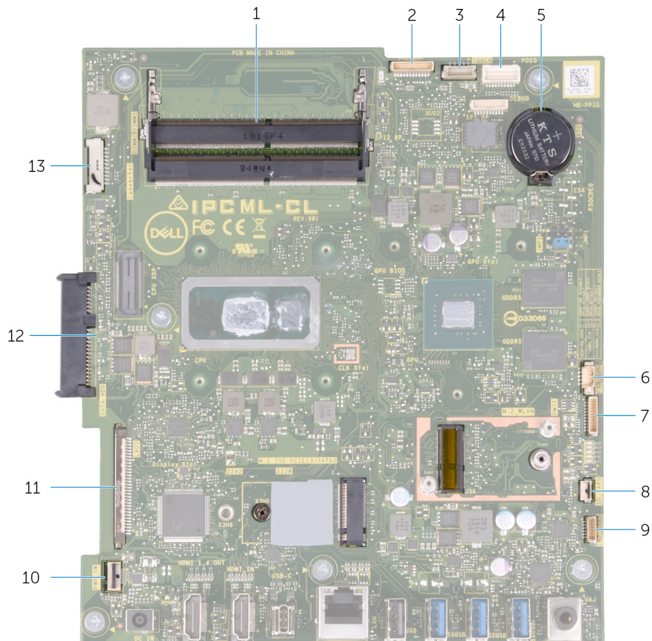
Afbeelding 1. Systeemkaartconnectoren.
