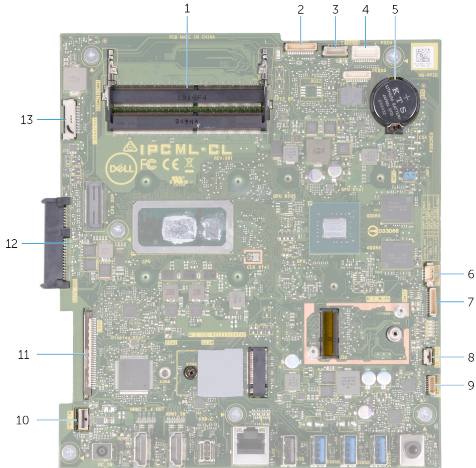
1. ábra. Alaplapi csatlakozók
