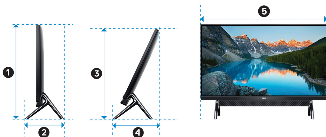
3. táblázat: Kétlábú állvány méretei
