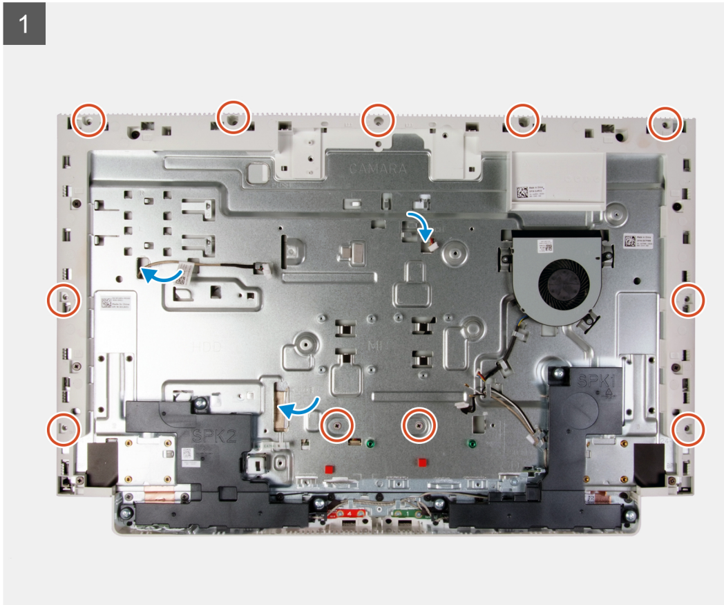
11x M3x5
