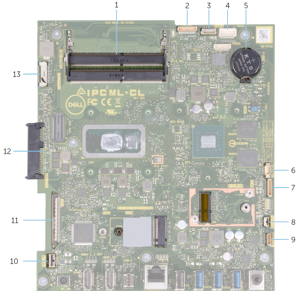
図 1. システム基板のコネクタ
