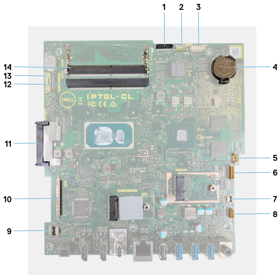
Rysunek 1. Złącza płyty głównej
