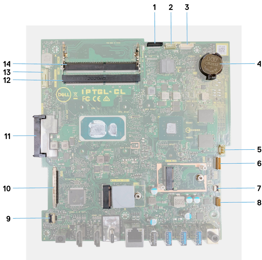
Figura 1. Connettori della scheda di sistema
