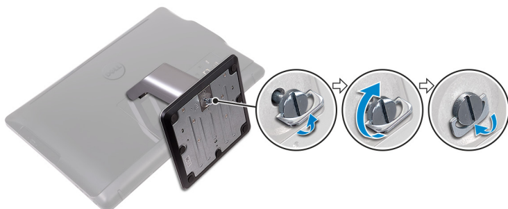
Рисунок 3. Затяжка невыпадающего винта для крепления основания к подставке
