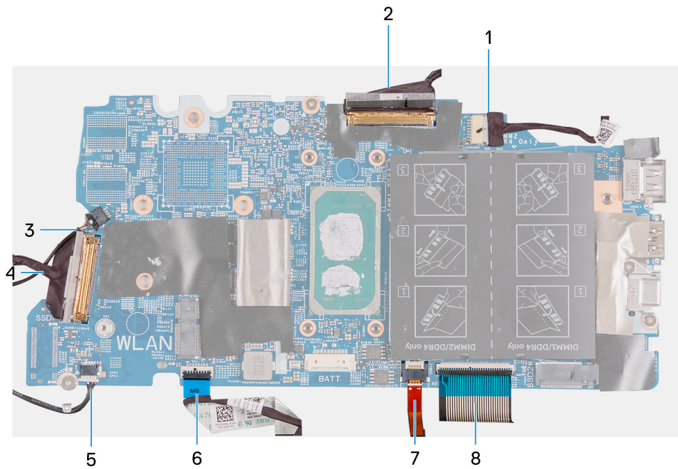
Abbildung 1. Systemplatineanschlüsse
