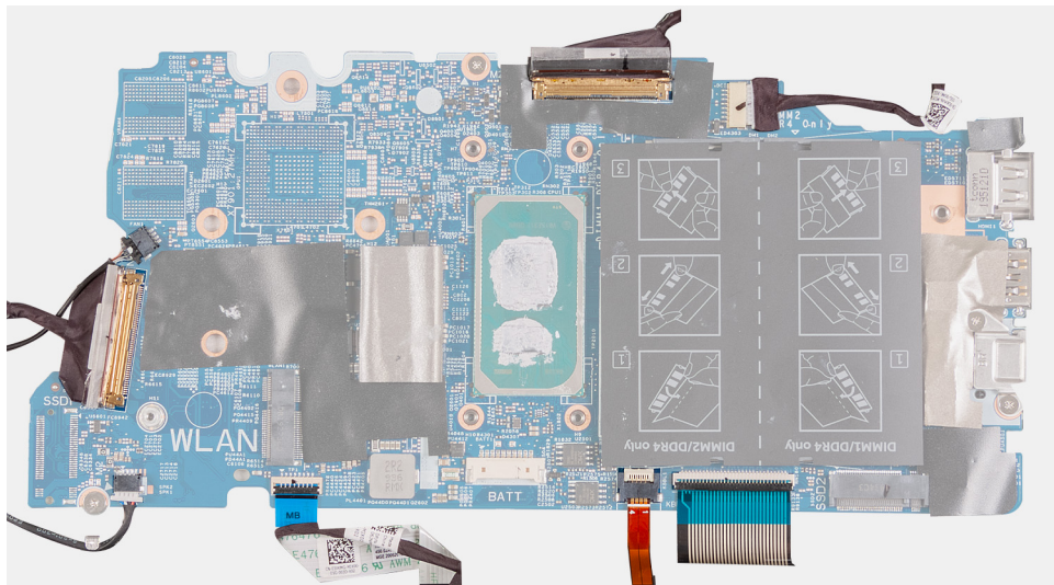
Abbildung 2. Systemplatinenanschlüsse
