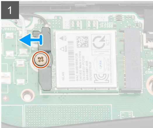
1x M2x4
