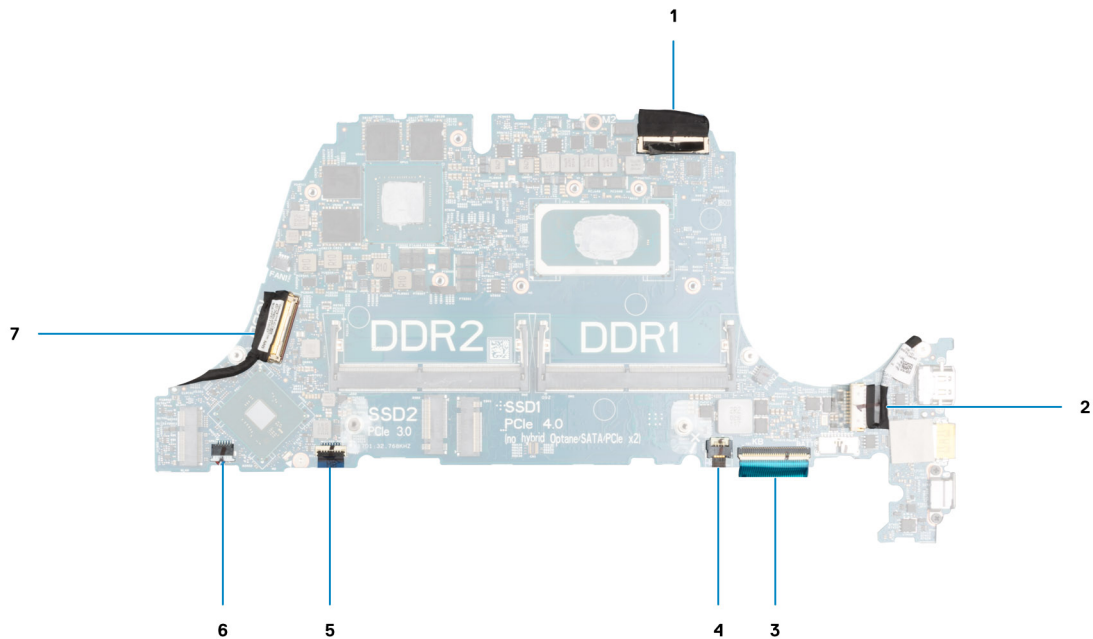
그림 2. 시스템 보드 커넥터
