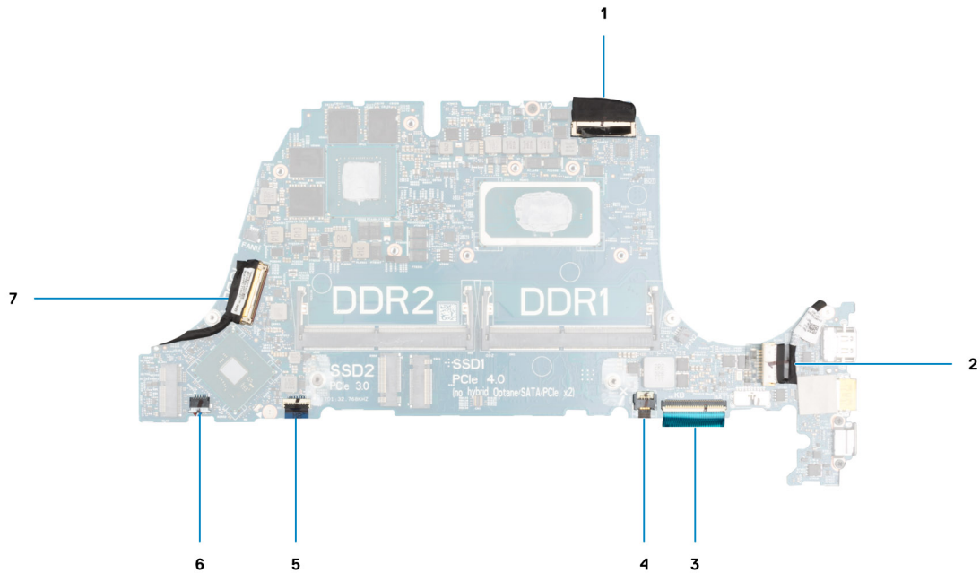
그림 1. 시스템 보드 커넥터
