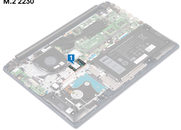
M.2 2230
