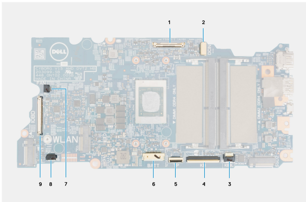
Abbildung 1. Systemplatinenanschlüsse
