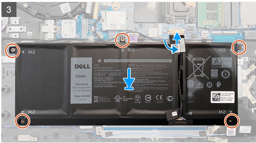
5x M2x3
