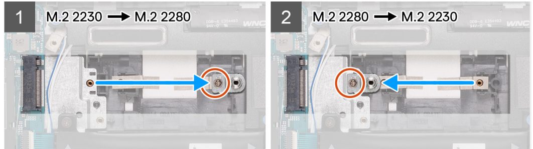
1x M1.6x2.5
