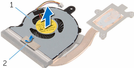
1 fan
