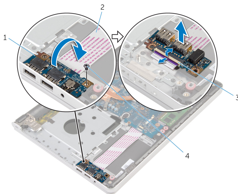
2. I/O 板纜線
