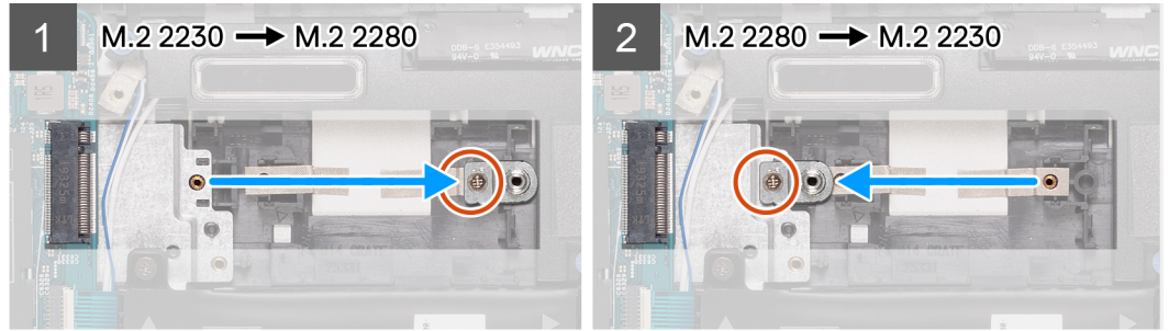
1x M1.6x2
