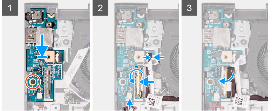
1x M2x3
