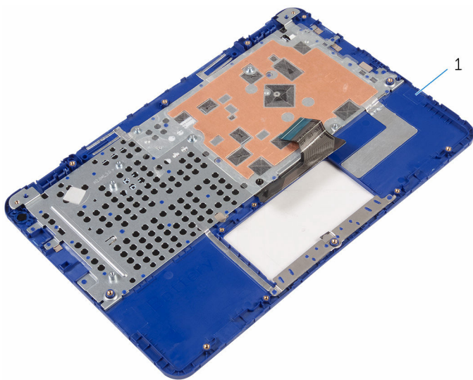
1 손목 받침대 및 키보드 조립품
