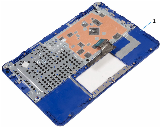
מכלול משענת כף היד והמקלדת 1
