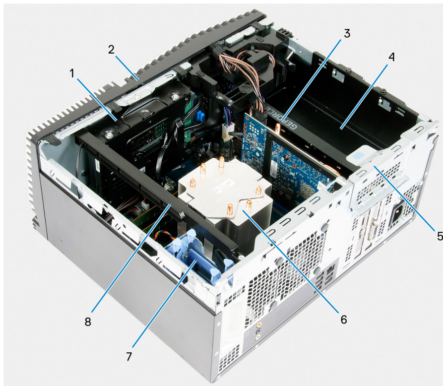
Figure 1. Vue intérieure de l'ordinateur
