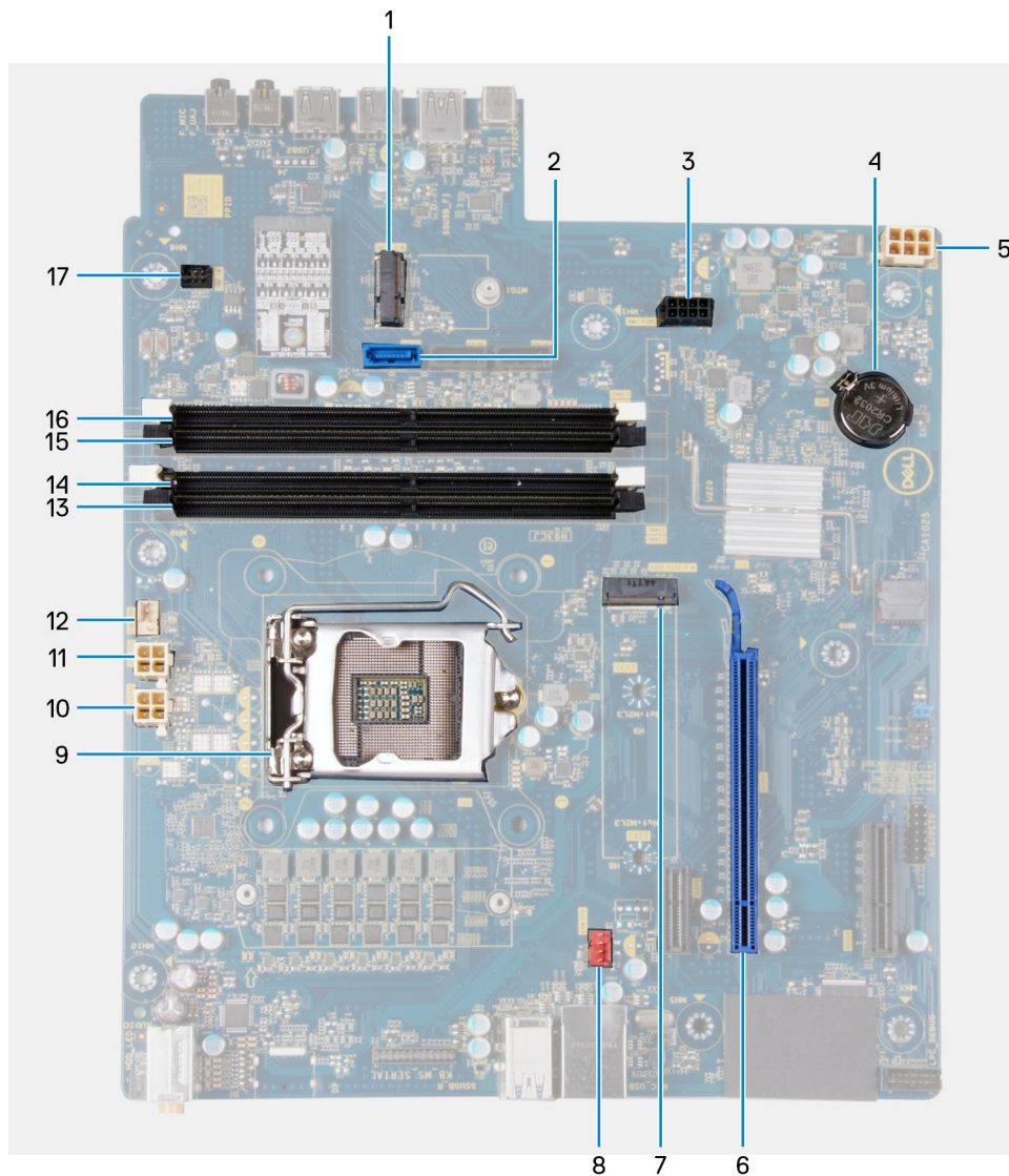
Figure 3. Composants de la carte système
