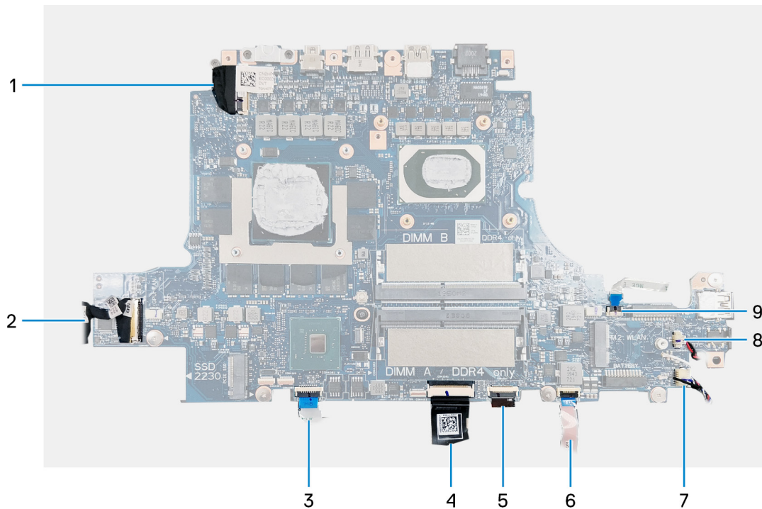
Figur 1. Hovedkortkabler
