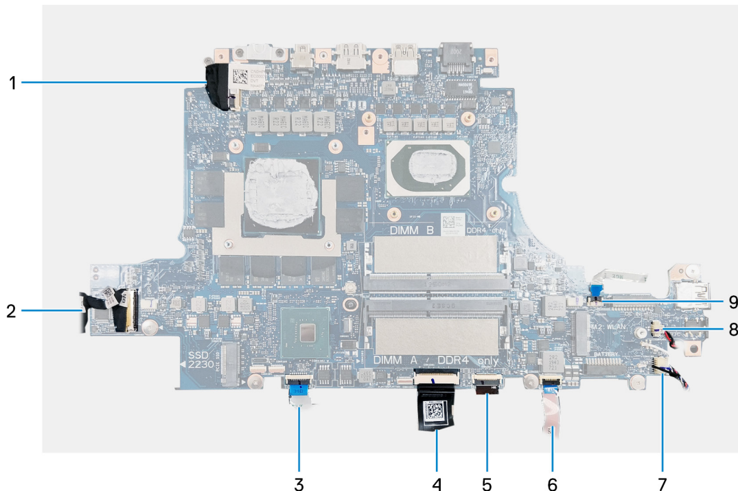
Figure 1. Câbles de la carte système
