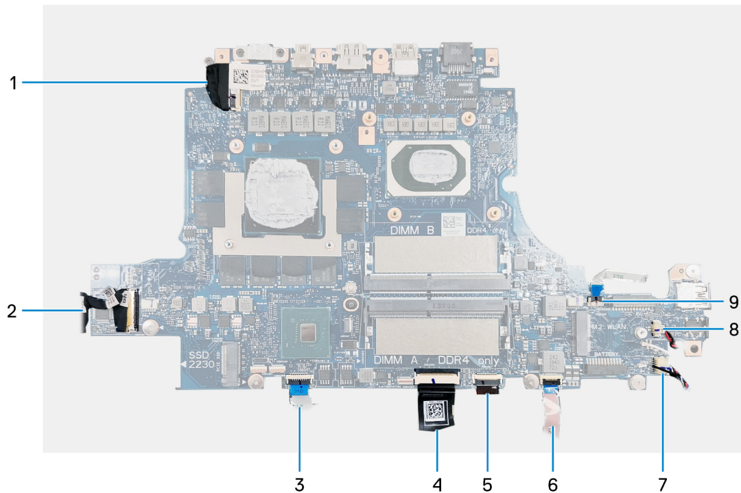
Figure 2. Câbles de la carte système
