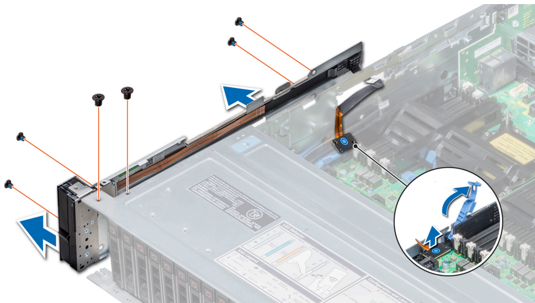
图 75: 卸下左侧控制面板
