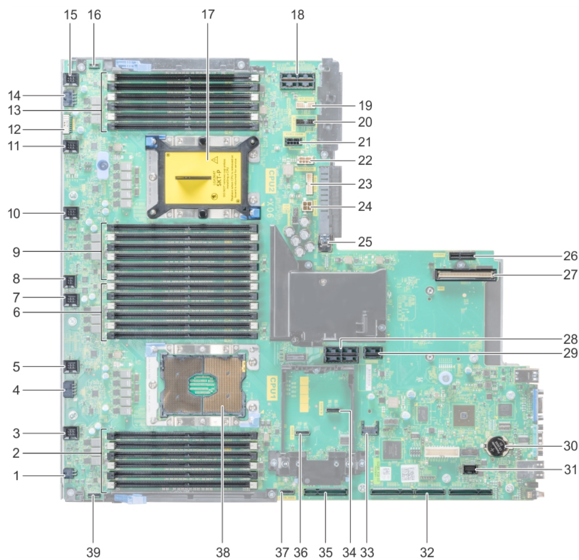
图 79: 系统板跳线和连接器
