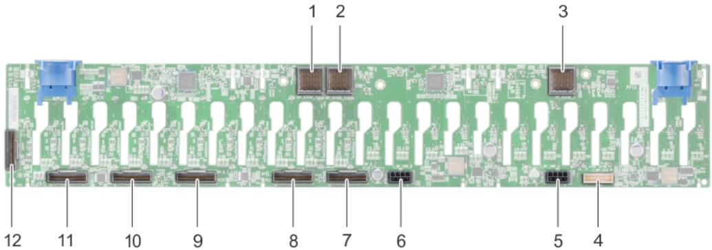
图 64: 24 x 2.5 英寸背板的背面视图
