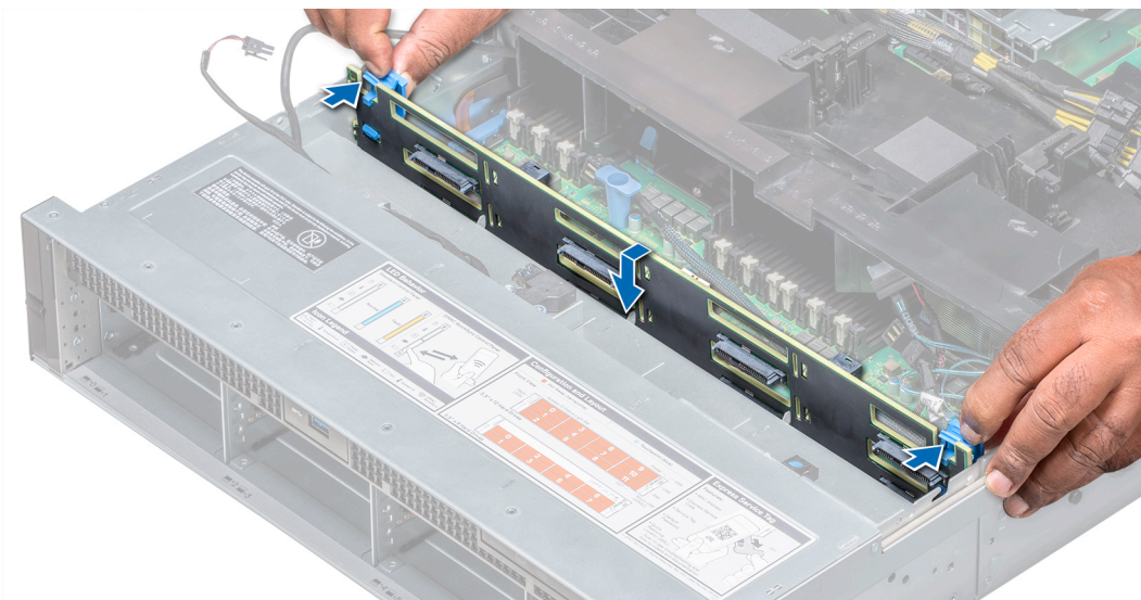
图 67: 安装硬盘驱动器背板
