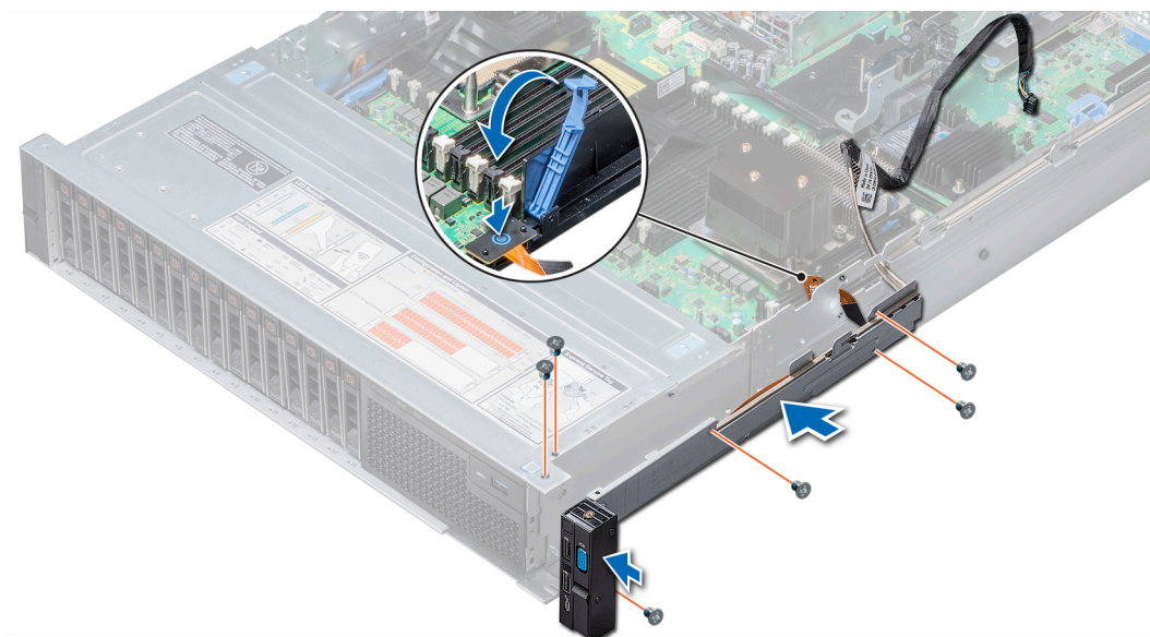
图 78: 安装右控制面板
