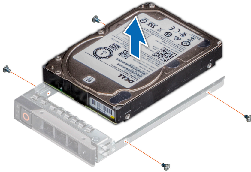
图 34: 从硬盘驱动器托盘中卸下硬盘驱动器
