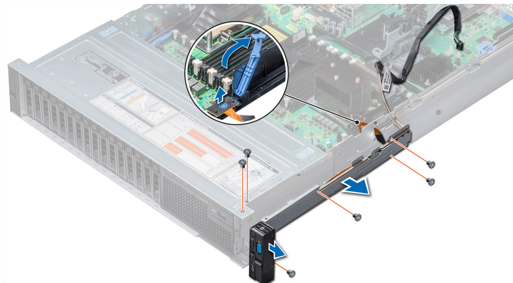
图 77: 卸下右侧控制面板
