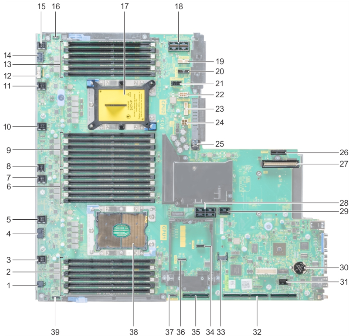
Abbildung 79. Jumper und Anschlüsse auf der Systemplatine
