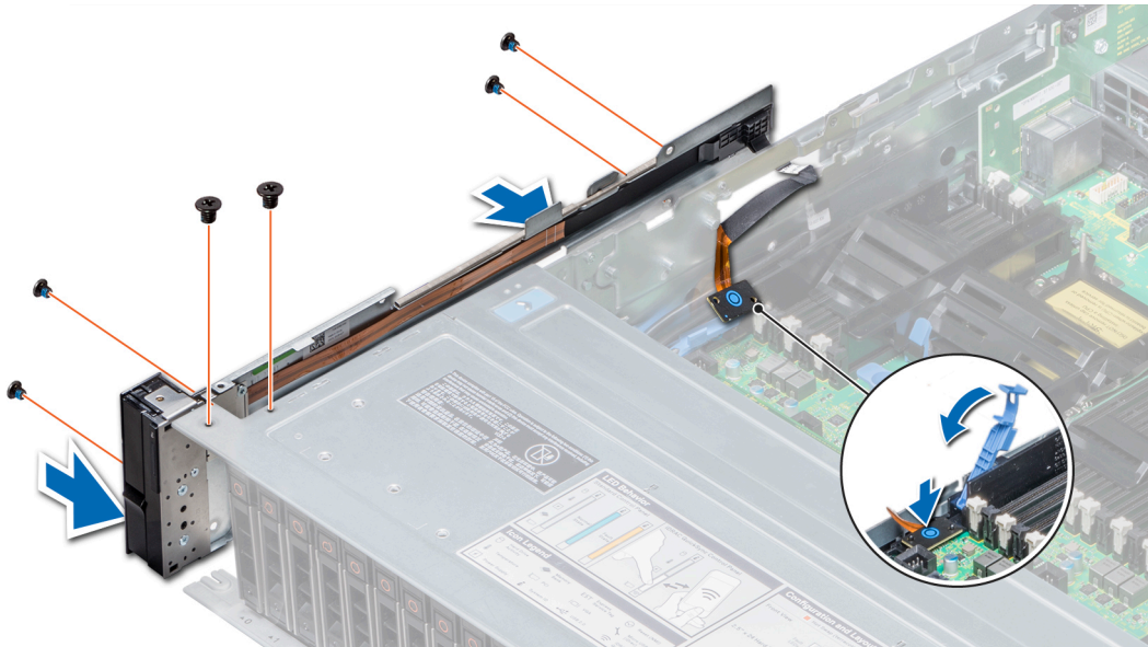
Abbildung 76. Installieren der Kabelabdeckung
