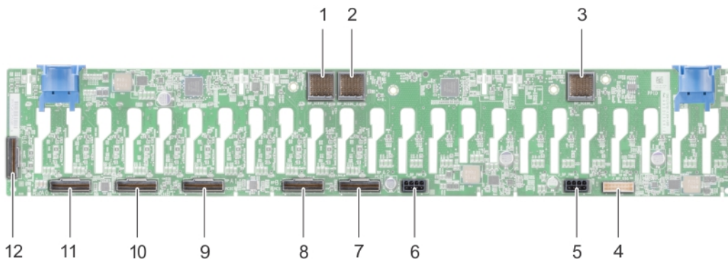
Abbildung 64. Rückansicht der 24 x 2,5-Zoll-Rückwandplatine
