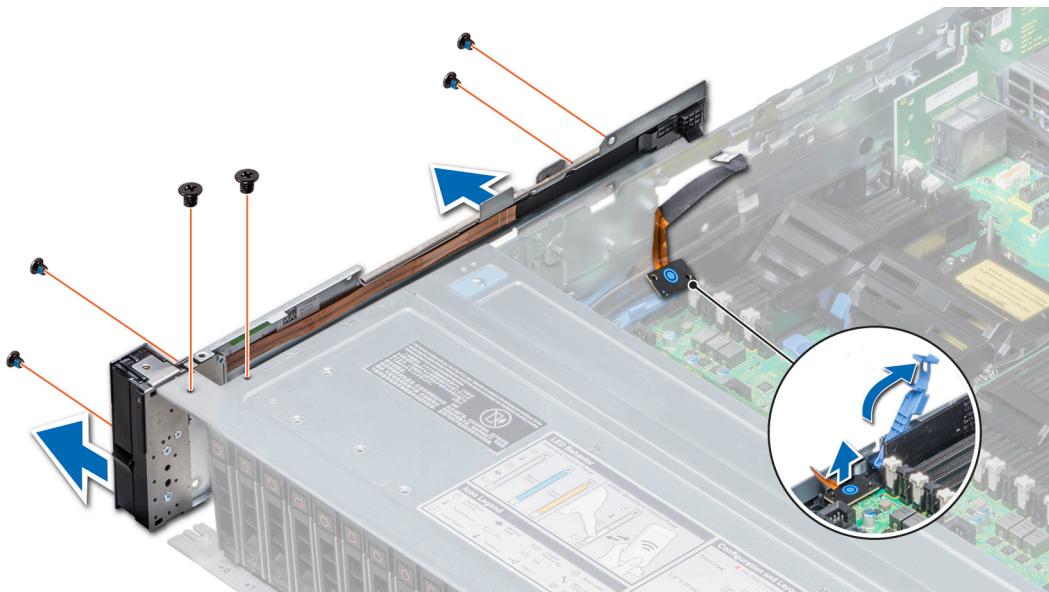
Abbildung 75. Entfernen des linken Bedienfelds
