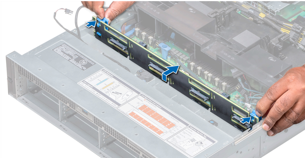
Abbildung 66. Entfernen der Festplatten-Rückwandplatine
