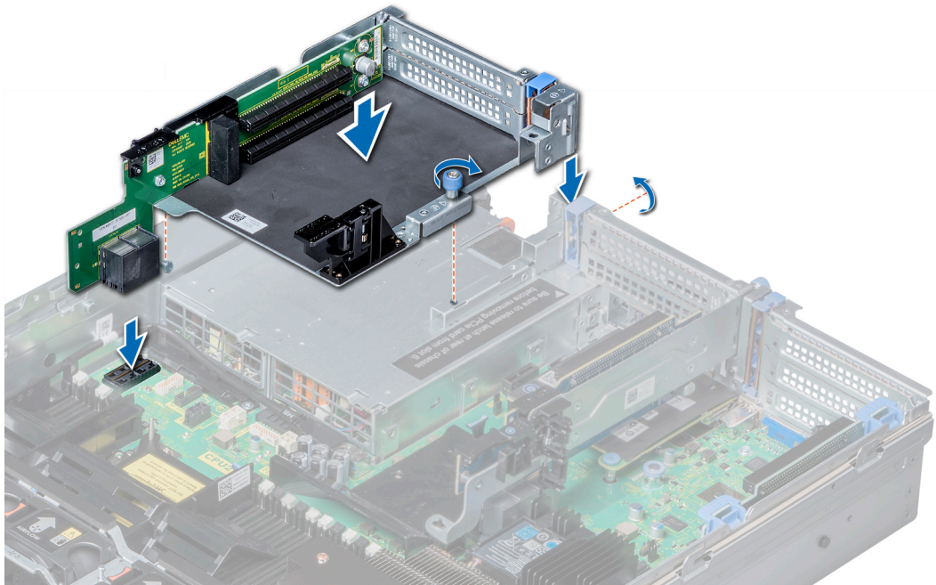
Abbildung 58. Einsetzen eines Erweiterungskarten-Risers 3
