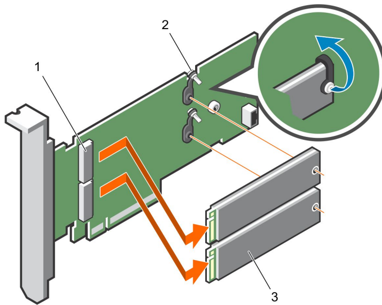
Abbildung 83. Entfernen des M.2 SSD-Moduls
