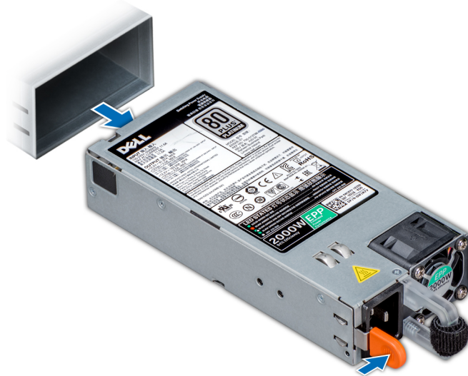
Abbildung 70. Entfernen einer Netzteilereinheit
