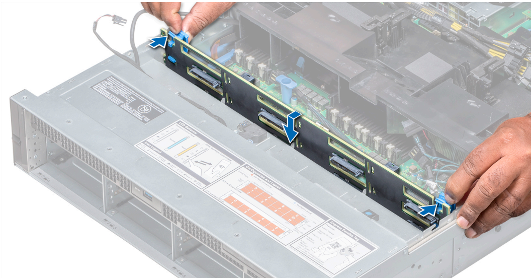
Abbildung 67. Installieren der Festplatten-Rückwandplatine
