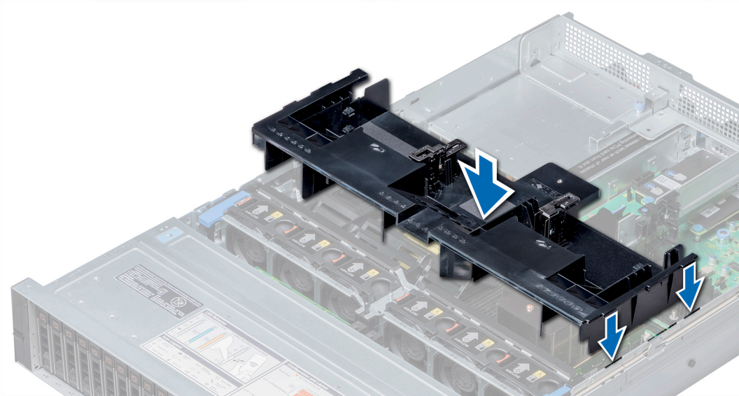
Abbildung 23. Installieren des Kühlgehäuses
