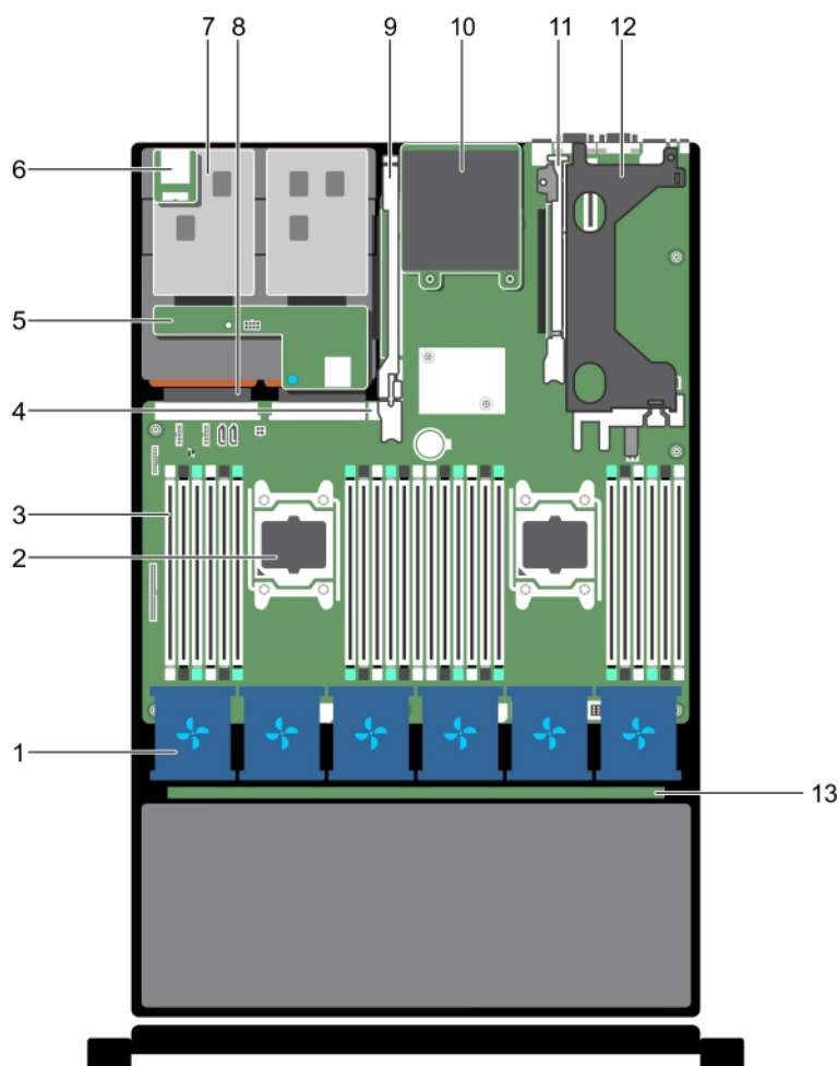
Ilustración 11. Interior del sistema: Dell XC730xd-12C
