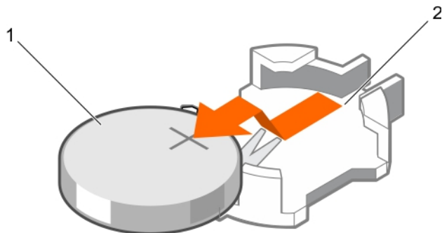
Ilustración 39. Extracción de la batería del sistema
