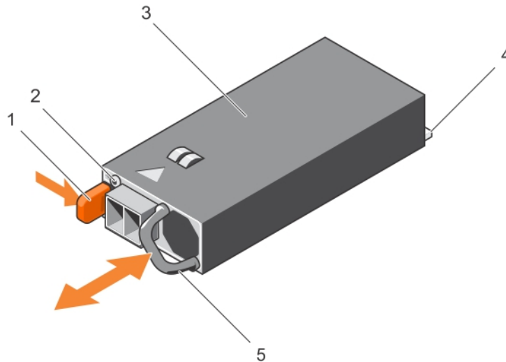
Ilustración 43. Extracción e instalación de una fuente de alimentación de CC
