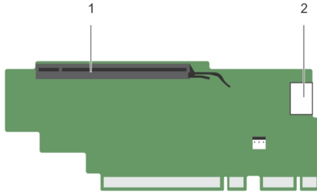
Ilustración 36. Identificación de los conectores del soporte vertical 3 para tarjetas de expansión (alternativo)
