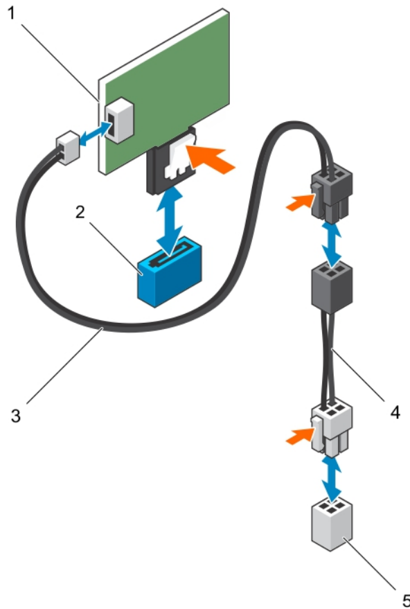
Ilustración 18. Extracción e instalación de SATADOM
