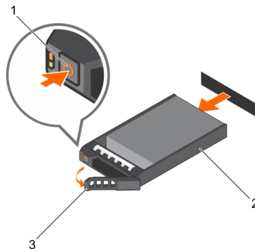
Ilustración 47. Extracción e instalación de una unidad de disco duro de intercambio directo
