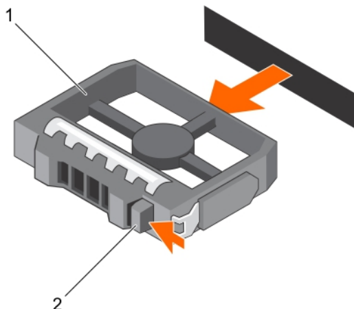
Ilustración 46. Extracción e instalación de una unidad de disco duro de relleno de 3,5 pulgadas
