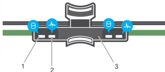
Ilustración 3. Indicadores HDD en el plano posterior de la bandeja de la unidad de disco duro
