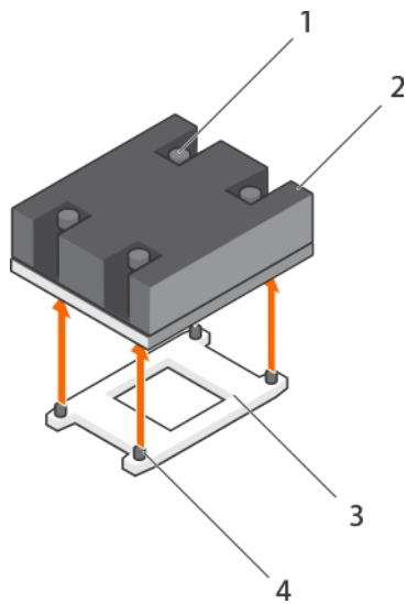
Ilustración 21. Extracción e instalación del disipador de calor del procesador
