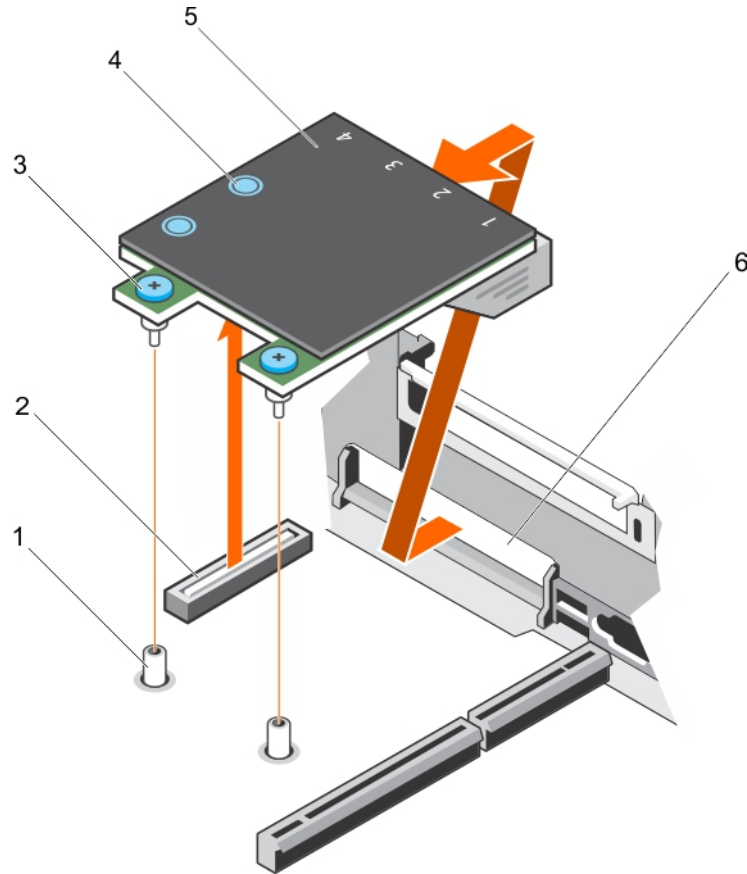
Ilustración 38. Extracción e instalación de la tarjeta secundaria de red (NDC)
