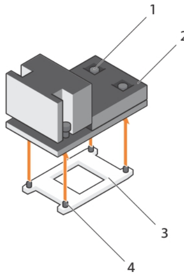
Ilustración 20. Extracción e instalación del disipador de calor del procesador
