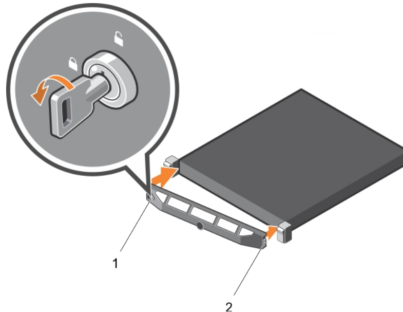
Ilustración 9. Extracción e instalación del embellecedor frontal
