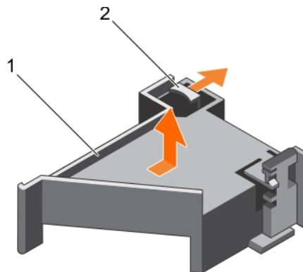
Ilustración 25. Extracción e instalación del soporte de tarjeta PCIe
