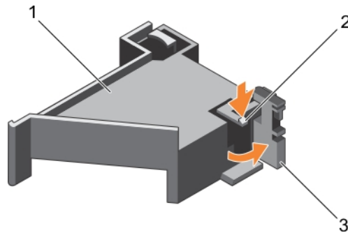
Ilustración 26. Apertura y cierre del pestillo del soporte de tarjeta PCIe
