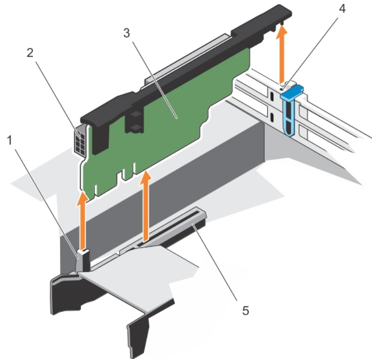
Ilustración 34. Extracción e instalación del soporte vertical 3 para tarjetas de expansión
