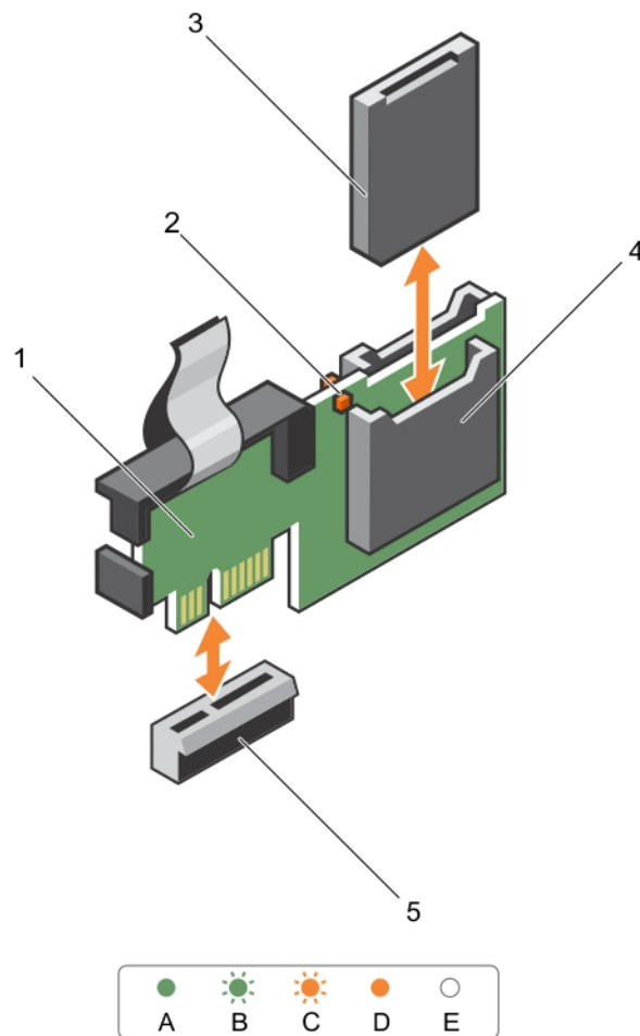
Ilustración 37. Extracción e instalación del módulo SD dual interno (IDSDM)
