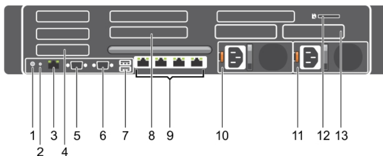
Ilustración 5. Características e indicadores del panel posterior
