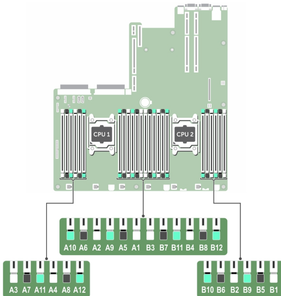
Ilustración 15. Ubicaciones de los zócalos de memoria
