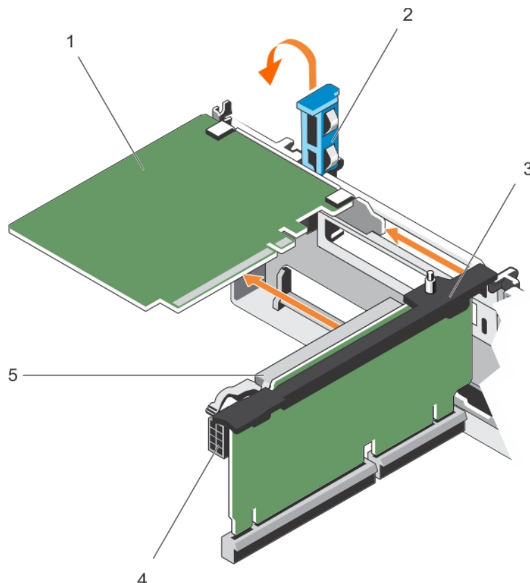
Ilustración 29. Extracción e instalación de una tarjeta de expansión de la tarjeta vertical de expansión 2 o 3
