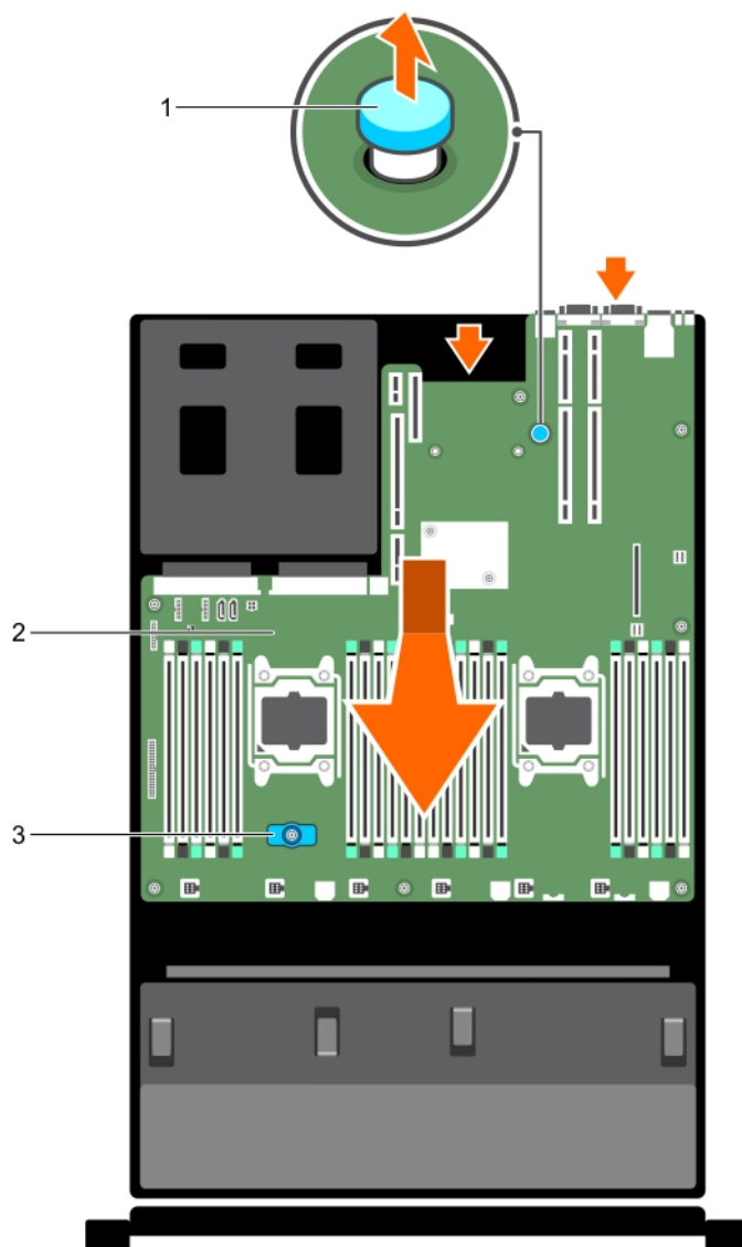
Ilustración 44. Extracción e instalación de la placa base
