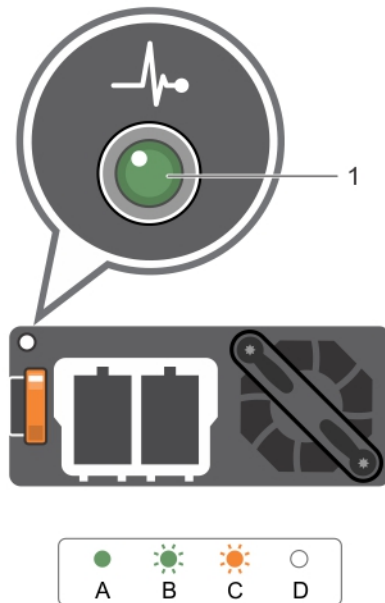
Ilustración 8. Indicador de estado de la unidad de fuente de alimentación de CC
