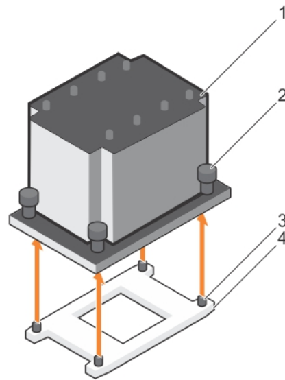
Ilustración 19. Extracción e instalación de un procesador
