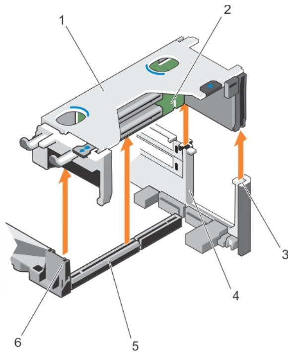
Ilustración 30. Extracción e instalación del soporte vertical 1 para tarjetas de expansión
