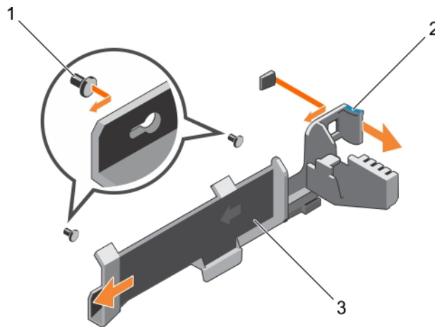
Ilustración 27. Extracción e instalación del soporte de retención de cables
