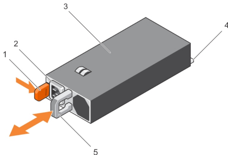
Ilustración 42. Extracción e instalación de una unidad de suministro de energía de CA
