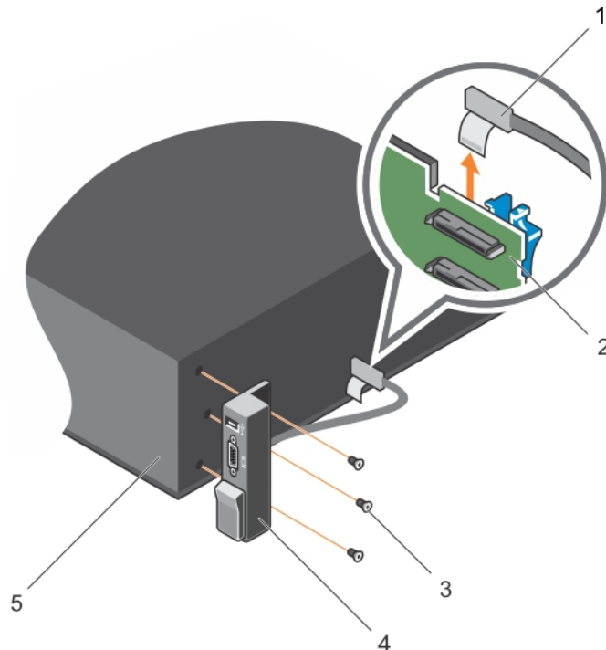
Ilustración 51. Extracción e instalación del panel de E/S
