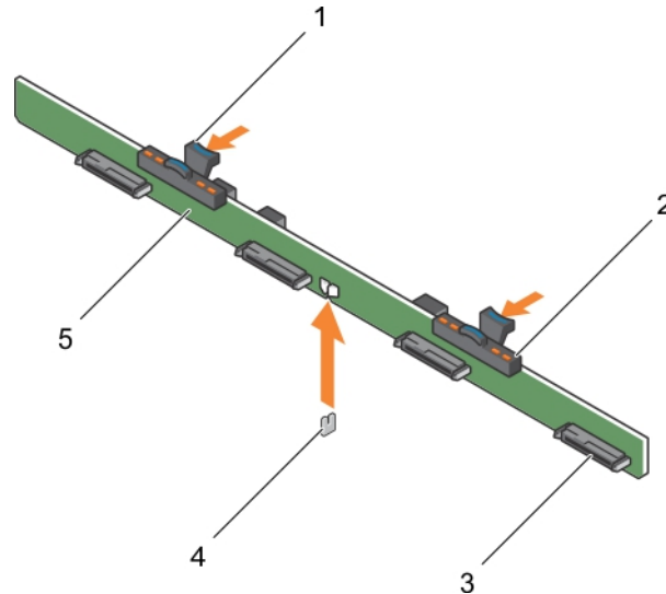
Ilustración 52. Extracción e instalación del plano posterior de la unidad de disco duro (x4) de 3,5 pulgadas
