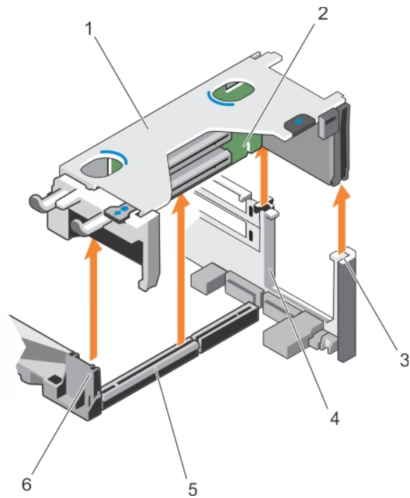
Abbildung 30. Entfernen und Einsetzen des Erweiterungskarten-Risers 1
