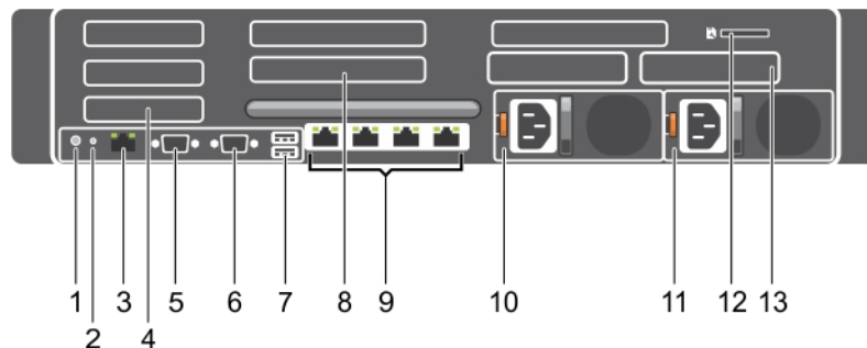
Abbildung 5. Funktionen und Anzeigen auf der Rückseite
