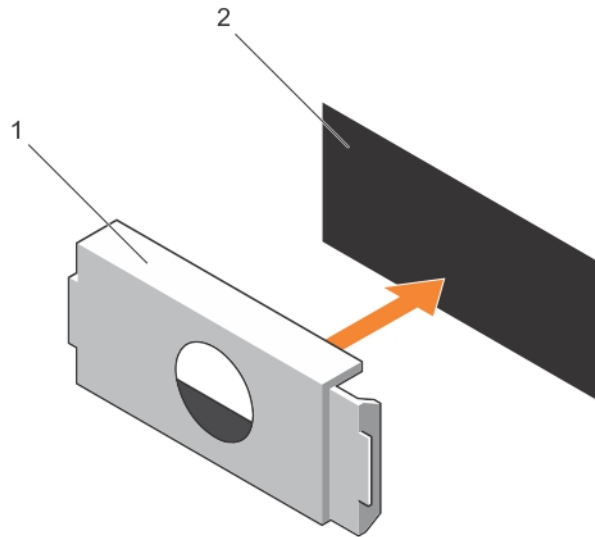
Abbildung 41. Entfernen und Einsetzen des Netzteilplatzhalters
