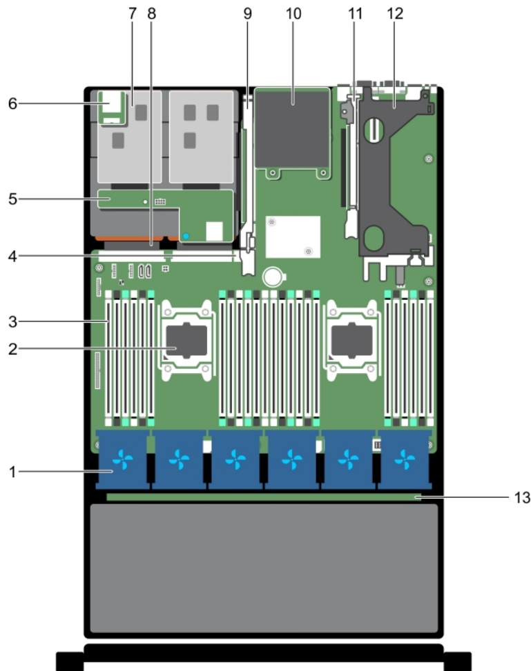
Abbildung 11. Das Innere des Systems – Dell XC730xd-12C
