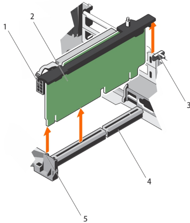
Abbildung 32. Entfernen und Einsetzen des Erweiterungskarten-Riser 2
