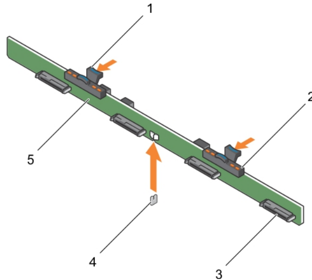
Abbildung 52. Entfernen und Installieren der 3,5-Zoll(x4)-Festplattenrückwandplatine
