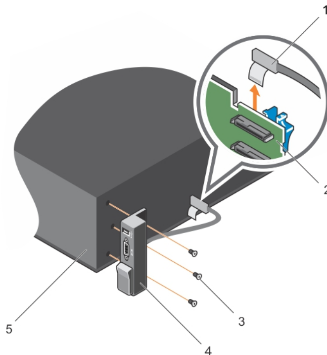
Abbildung 51. Entfernen und Installieren der E/A-Platine
