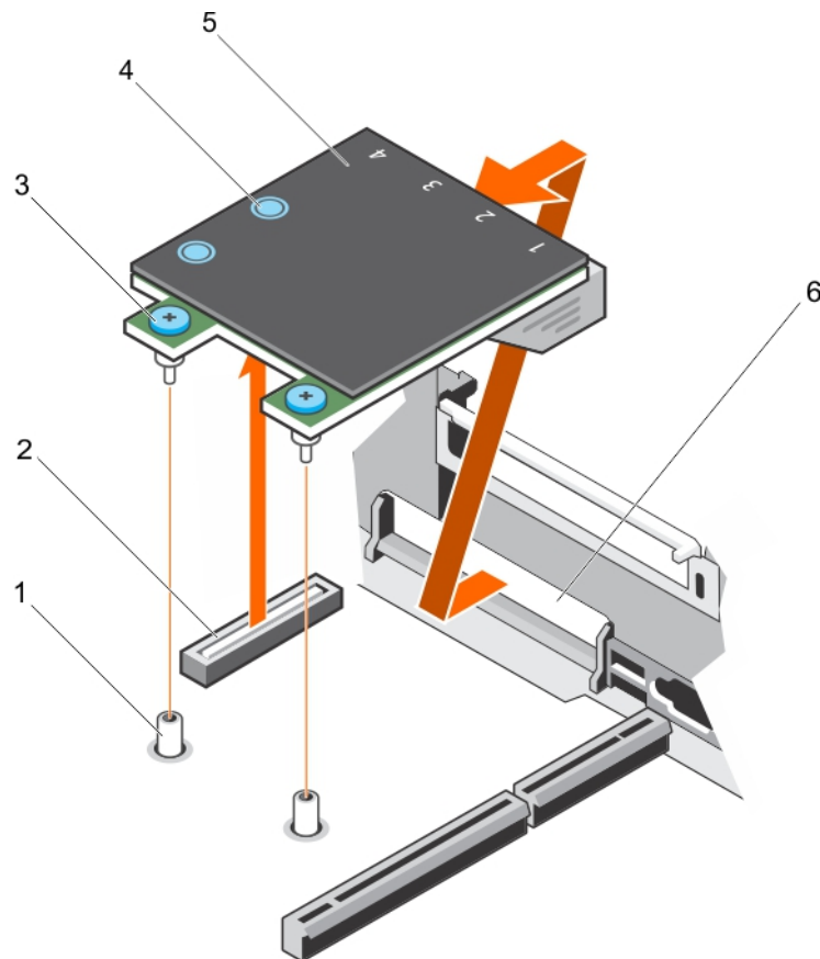
Abbildung 38. Entfernen und Einsetzen der Netzwerktochterkarte (NDC)
