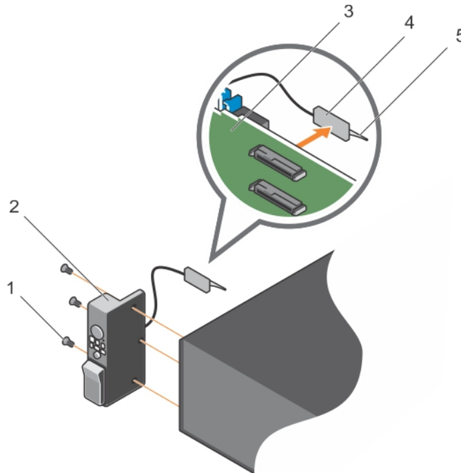
Abbildung 50. Entfernen und Installieren des Bedienfelds
