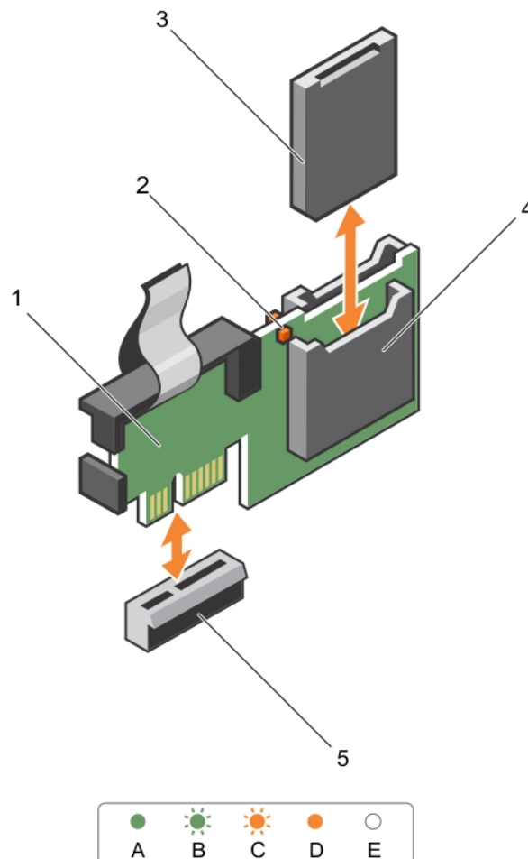
Abbildung 37. Entfernen und Einsetzen des internen Dual SD-Moduls (IDSDM)
