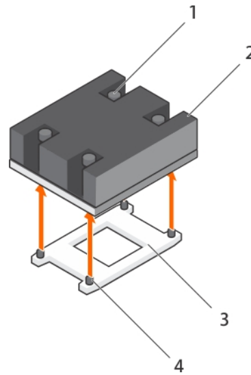
Abbildung 21. Entfernen und Einsetzen eines Prozessorkühlkörpers
