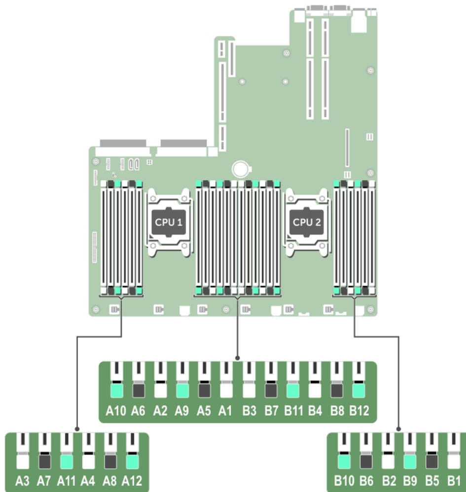
Abbildung 15. Positionen der Speichersteckplätze
