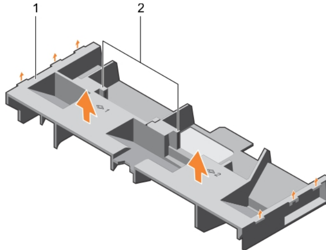
Abbildung 12. Entfernen und Einsetzen des Kühlgehäuses
