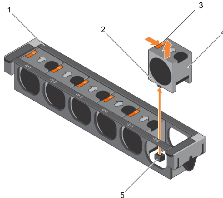
Abbildung 13. Entfernen und Installieren eines Kühlungsüfters
