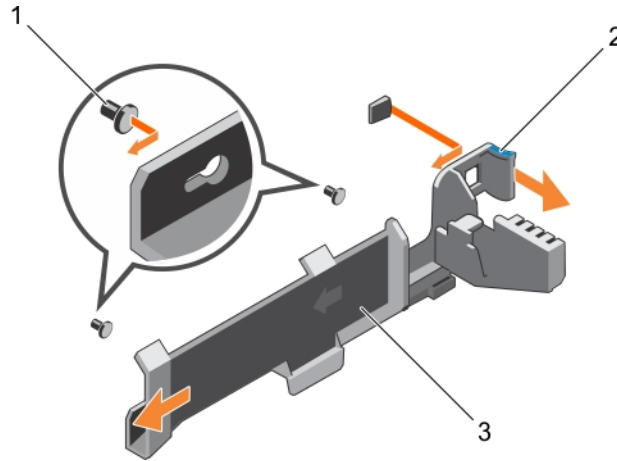
Abbildung 27. Entfernen und Einsetzen der Kabelhalteklammer
