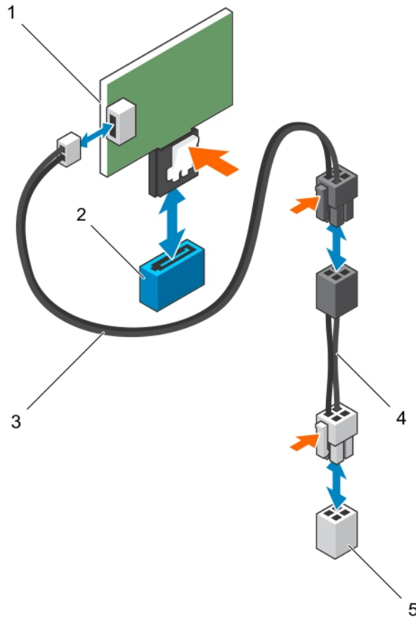
Abbildung 18. Entfernen und Installieren von SATADOM
