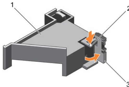
Abbildung 26. Öffnen und Schließen der PCIe-Kartenhalterverriegelung
