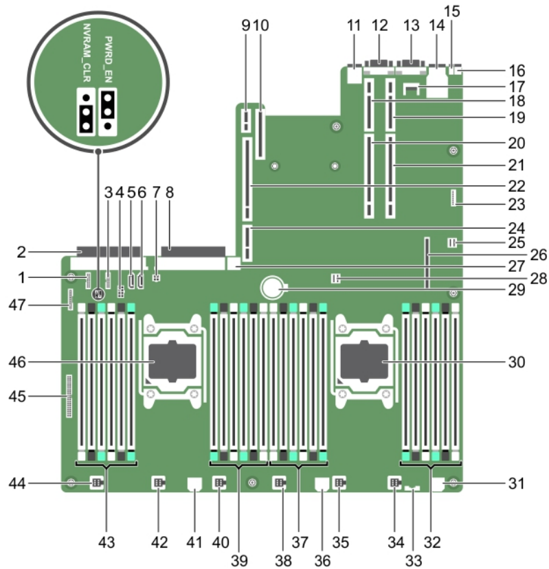
Abbildung 53. Jumper und Anschlüsse auf der Systemplatine
