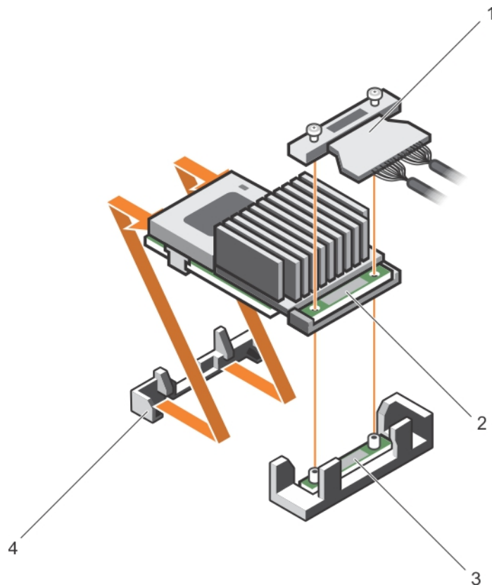
Abbildung 28. Entfernen und Einsetzen der integrierten Speichercontrollerkarte
