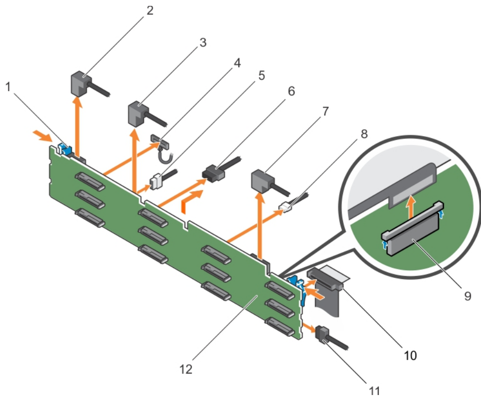
Abbildung 49. Entfernen und Installieren der 3,5-Zoll(x12)-SAS/SATA-Rückwandplatine
