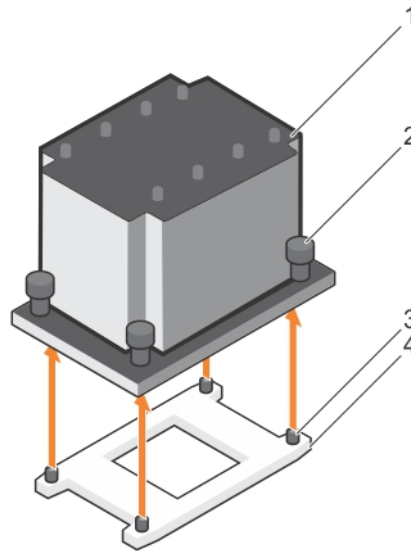
Abbildung 19. Entfernen und Einsetzen eines Prozessors
