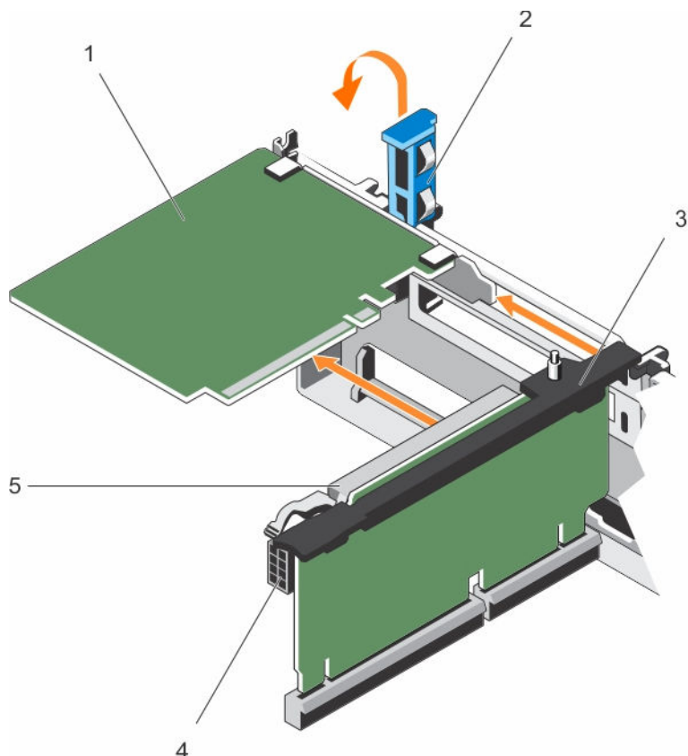
图 28: 在扩展卡提升板 2 或 3 中卸下和安装扩展卡
