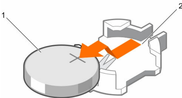
图 40: 卸下系统电池
