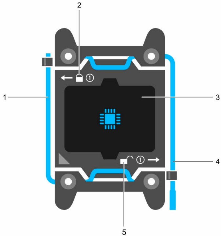
图 21: 处理器护罩
