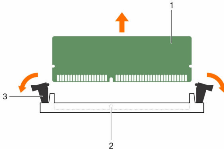
图 15: 卸下和安装内存模块
