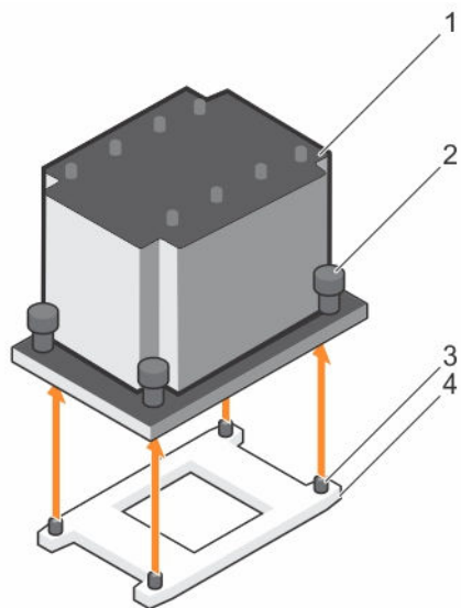
图 18: 卸下和安装处理器
