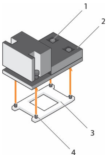
图 19: 卸下和安装处理器散热器
