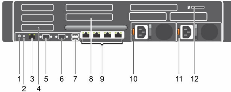
图 4: 背面板功能部件和指示灯
