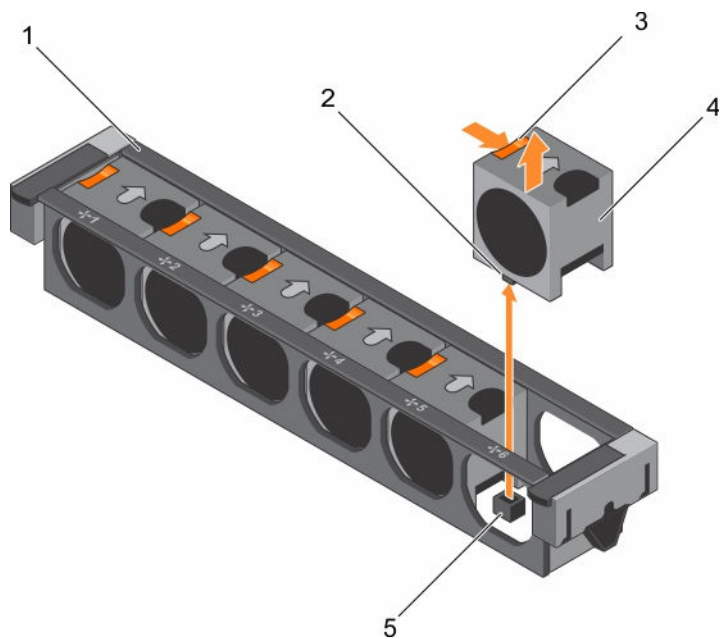
图 12: 卸下和安装冷却风扇
