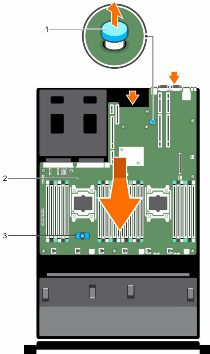
图 44: 卸下和安装系统板
