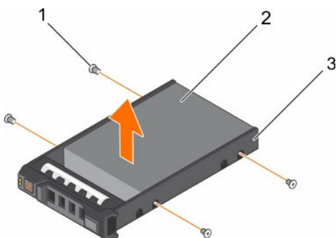
图 48: 在硬盘驱动器托架中卸下和安装硬盘驱动器
