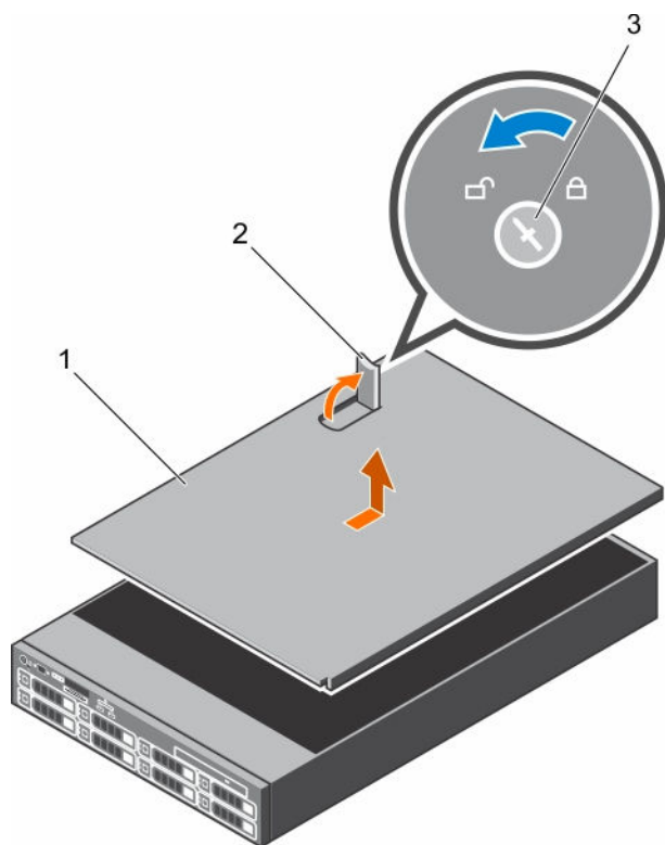
图 9: 卸下系统护盖
