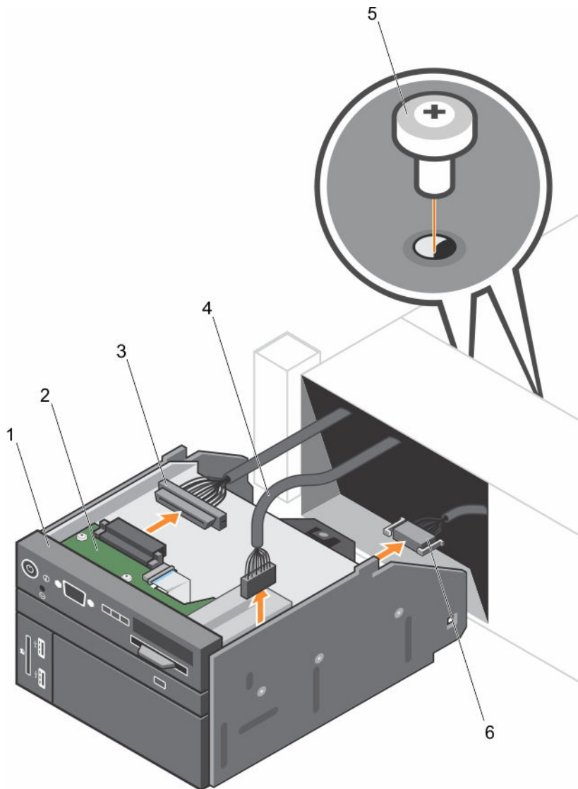
图 51: 卸下和安装控制面板
