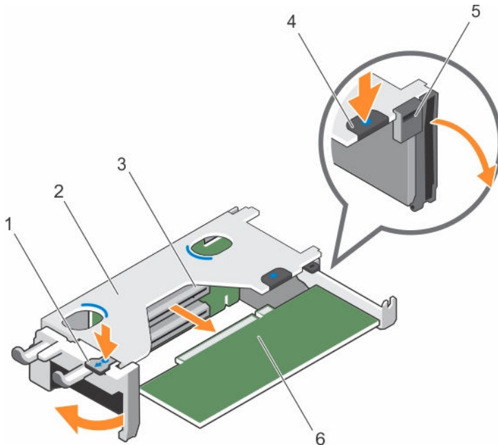
图 29: 在扩展卡提升板 1 中卸下和安装扩展卡
