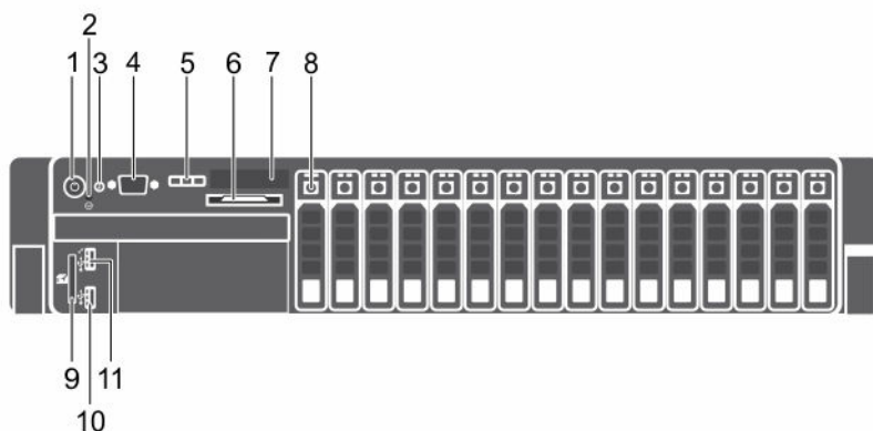
图 1: 前面板功能部件和指示灯
