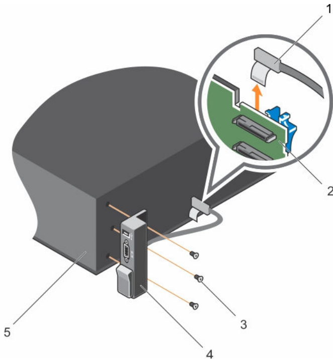
图 53: 卸下和安装 I/O 面板
