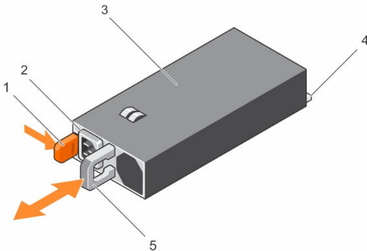
图 42: 卸下和安装交流电源设备
