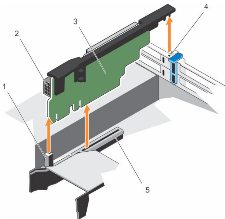
图 34: 卸下和安装扩展卡提升板 3
