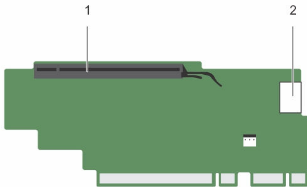
图 36: 识别扩展卡提升板 3 上的连接器（备用）
