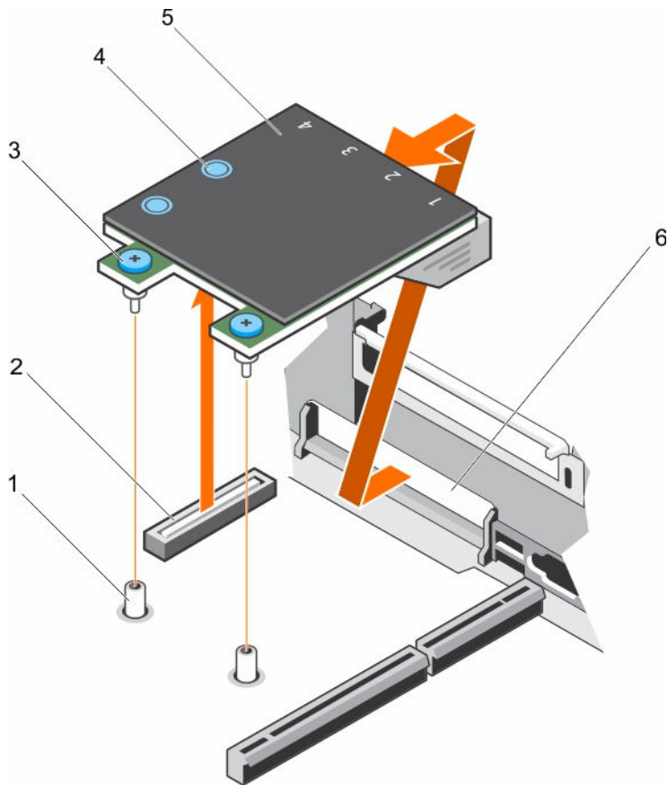
图 39: 卸下和安装网络子卡 (NDC)
