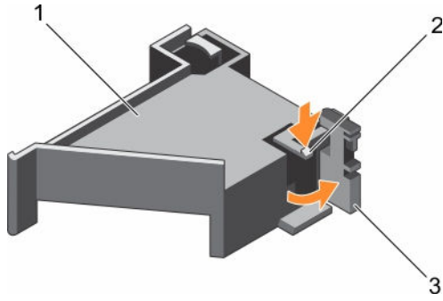
图 25: 打开和关闭 PCIe 卡固定器闩锁
