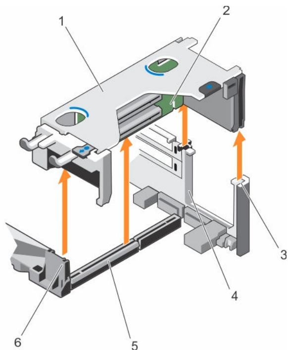
图 30: 卸下和安装扩展卡提升板 1
