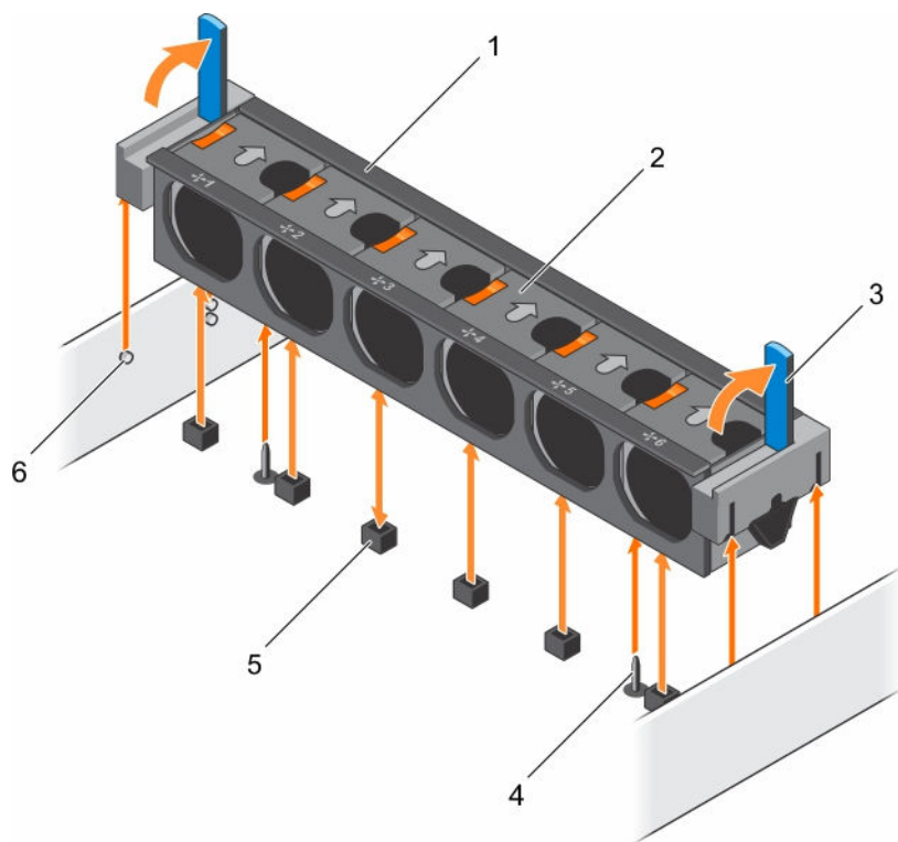
图 13: 卸下和安装冷却风扇部件
