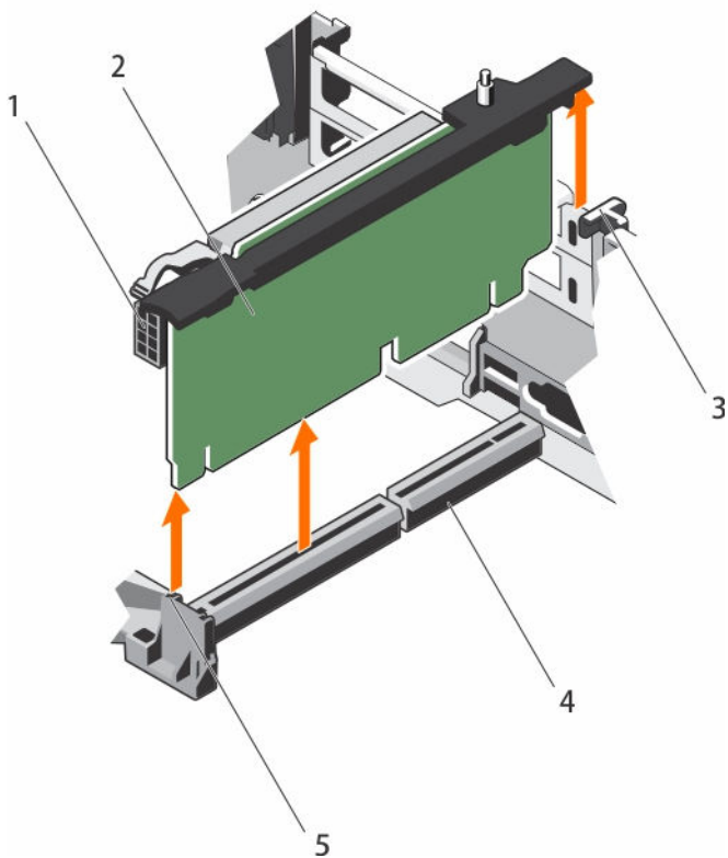
图 32: 卸下和安装扩展卡提升板 2
