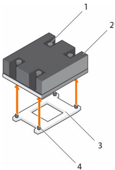
图 20: 卸下和安装处理器散热器
