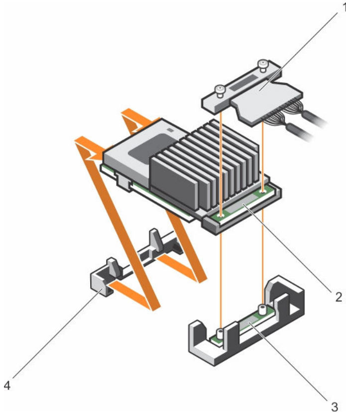
图 27: 卸下和安装集成存储控制器卡
