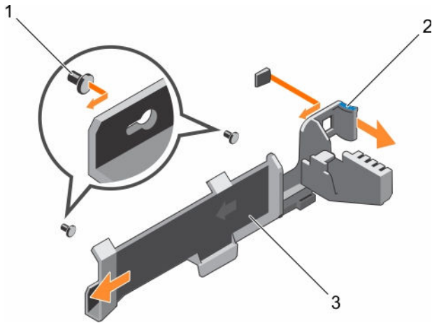
图 26: 卸下和安装电缆固定支架
