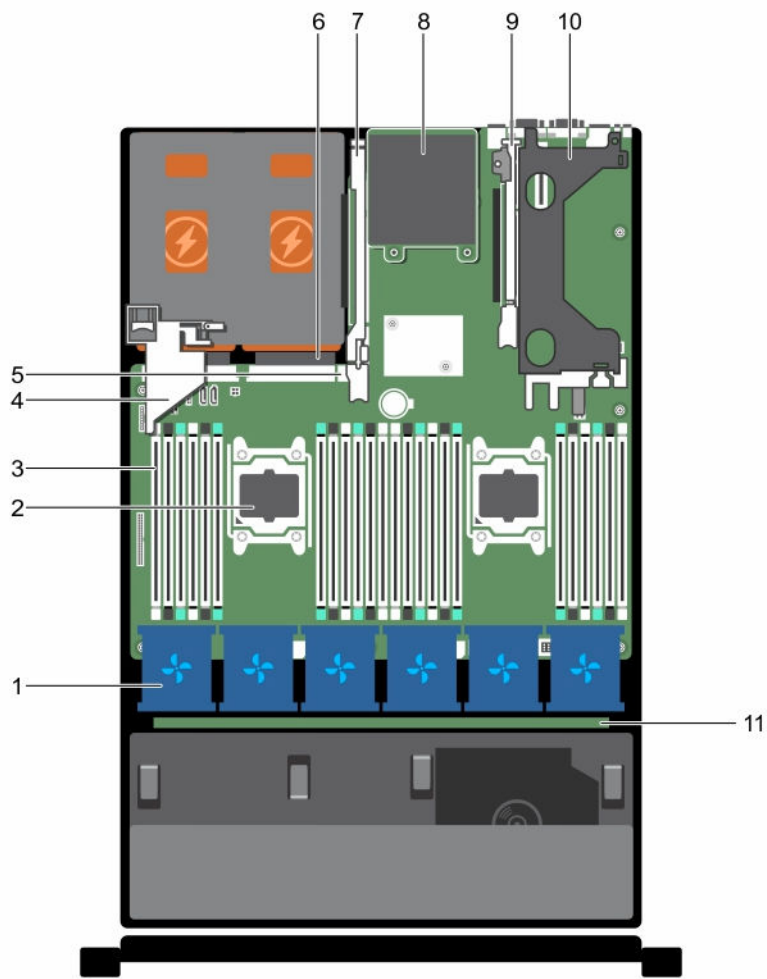
图 10: 系统内部 - Dell XC730-16G
