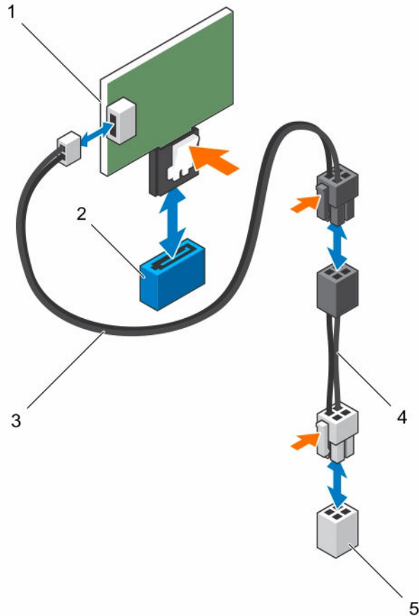
图 17: 卸下和安装 SATADOM
