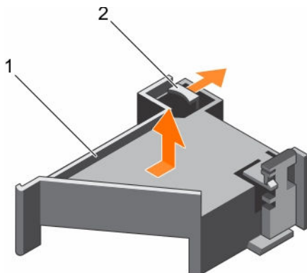
图 24: 卸下和安装 PCIe 卡固定器
