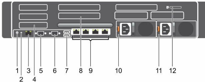
그림 4. 후면 패널 구조 및 표시등
