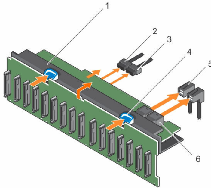
그림 49 . 2.5인치(x16) SAS/SATA 후면판 분리 및 설치
