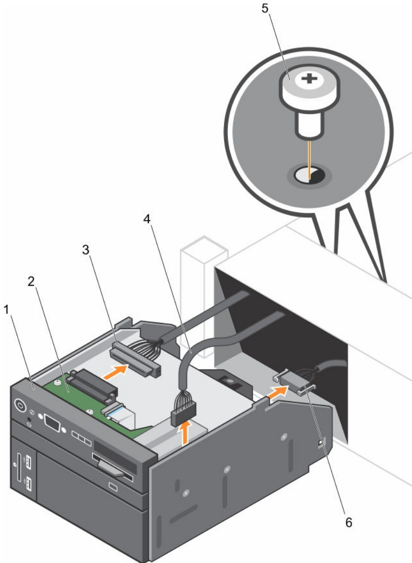
그림 51. 제어판 분리 및 설치
