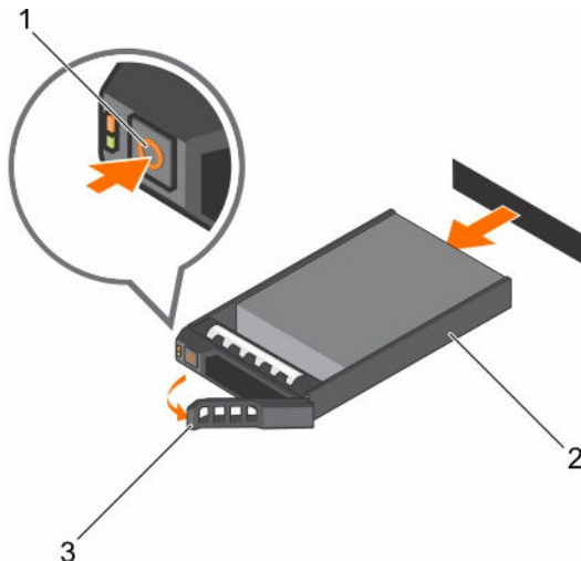
그림 47. 핫 스왑 하드 드라이브 분리 및 설치
