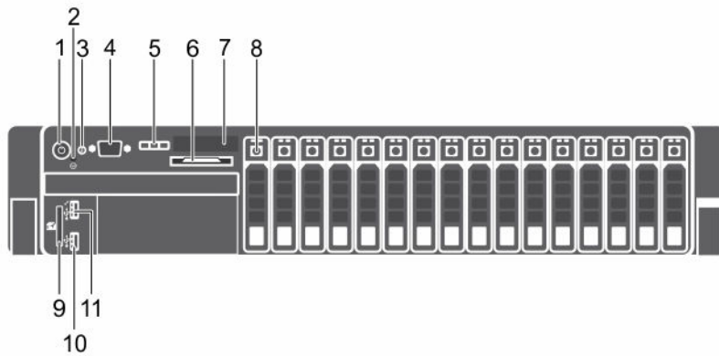
그림 1. 전면 패널 구조 및 표시등
