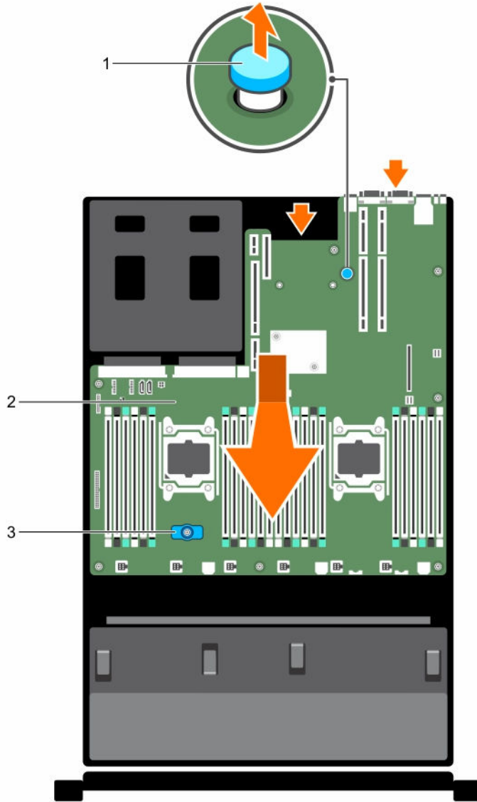
그림 44. 시스템 보드 분리 및 설치
