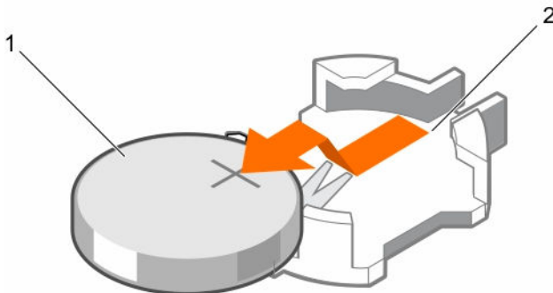
그림 40. 시스템 전지 분리
