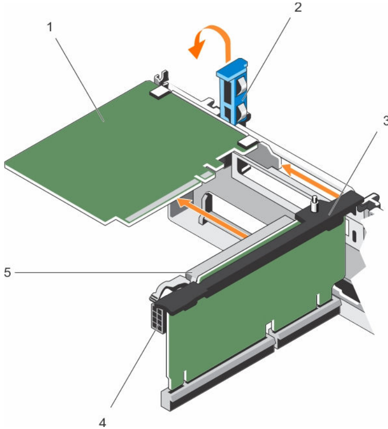
그림 28. 확장 카드 라이저 2 또는 3에서의 확장 카드 설치 및 분리
