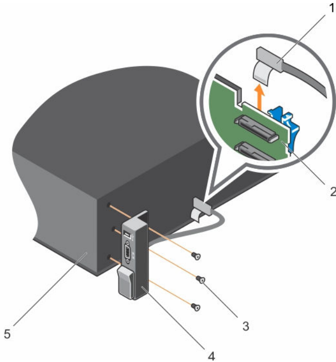
그림 53. I/O 패널 분리 및 설치
