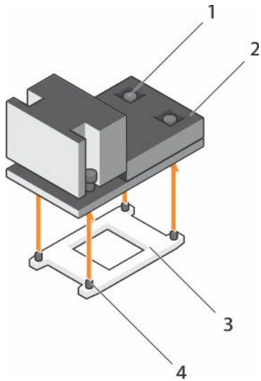
그림 19. 프로세서 방열판 분리 및 설치
