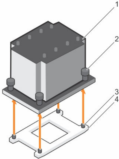
그림 18. 프로세서 분리 및 설치
