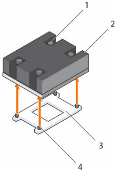
그림 20. 프로세서 방열판 분리 및 설치
