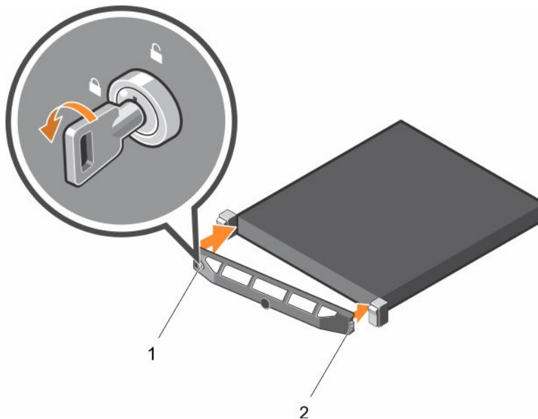
그림 8. 전면 베젤 분리 및 설치
