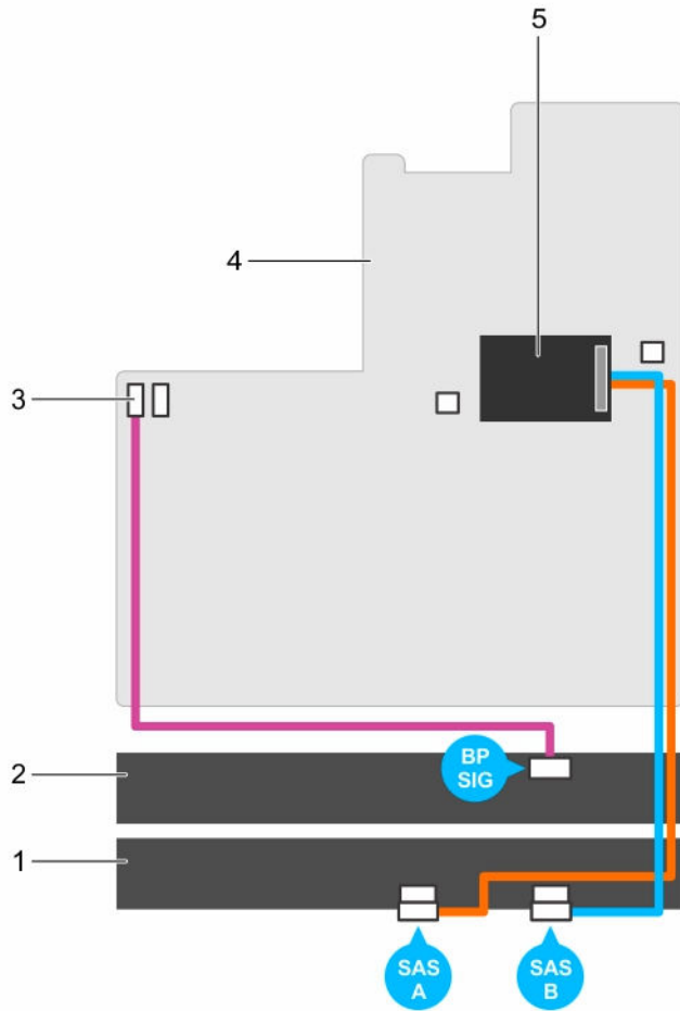
그림 50. 케이블 연결 - 2.5인치 (x16) SAS/SATA 후면판
