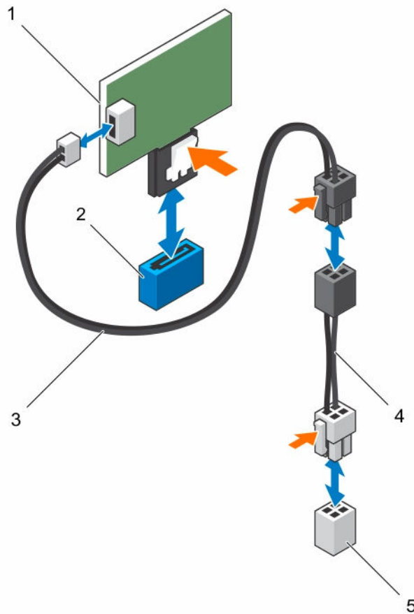
그림 17. SATADOM 분리 및 설치
