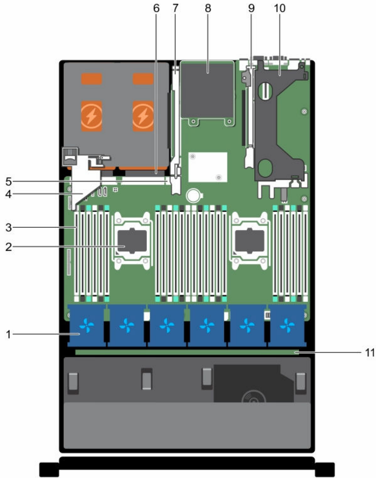
그림 10 . 시스템 내부 - Dell XC730-16G
