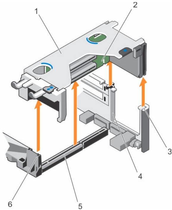
그림 30. 확장 카드 라이저 1 분리 및 설치
