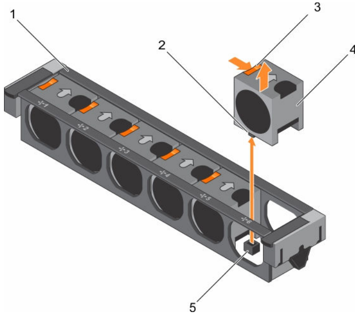
그림 12. 냉각 팬 분리 및 설치
