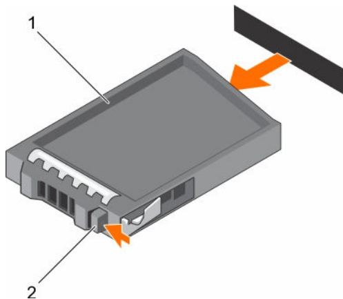
그림 46. 2.5인치 하드 드라이브 보호물 분리 및 설치
