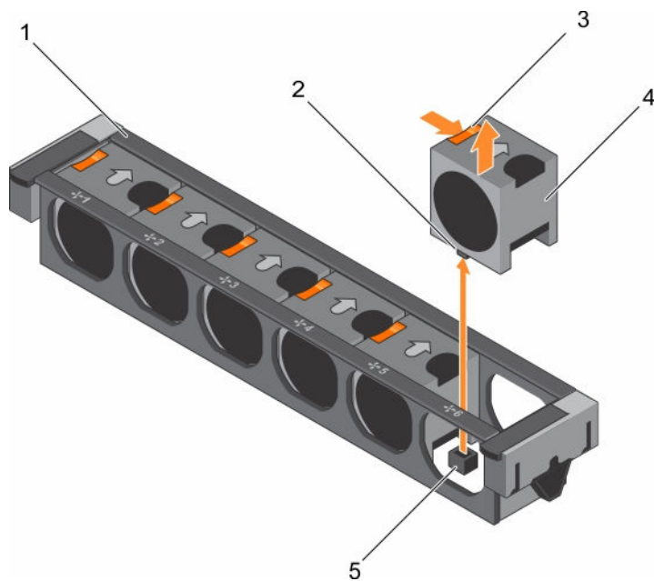
図 12. 冷却ファンの取り外しと取り付け
