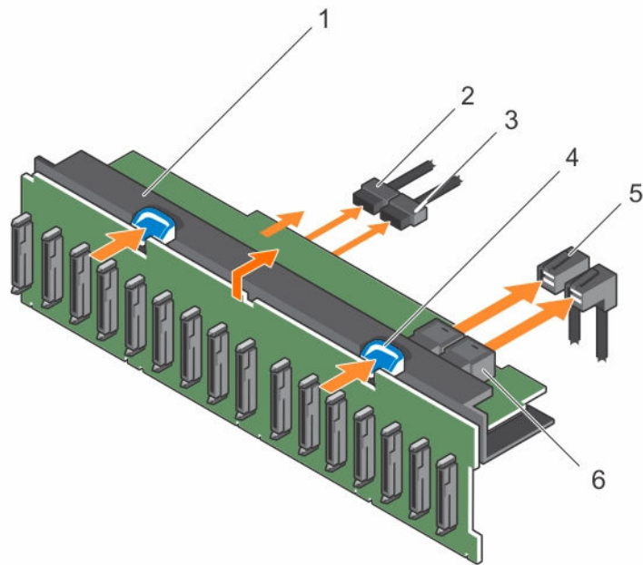
図 49. 2.5 インチ (x16) SAS/SATA バックプレーンの取り外しと取り付け
