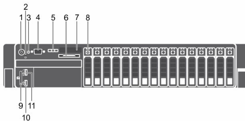
図 1. 前面パネルの機能とインジケータ
