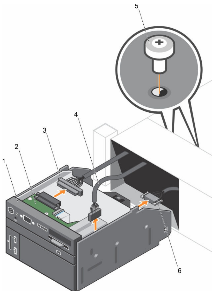
図 51. コントロールパネルの取り外しと取り付け
