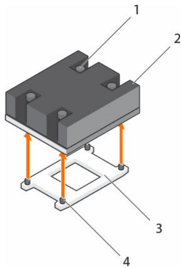
図 20. プロセッサヒートシンクの取り外しと取り付け
