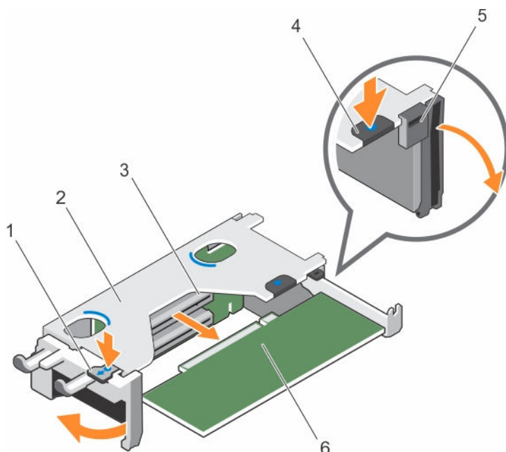
図 29. 拡張カードライザー 1 からの拡張カードの取り外しと取り付け
