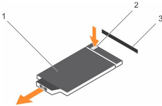
図 52. 情報タグの取り外しと取り付け
