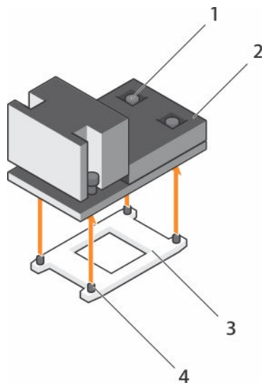
図 19. プロセッサヒートシンクの取り外しと取り付け
