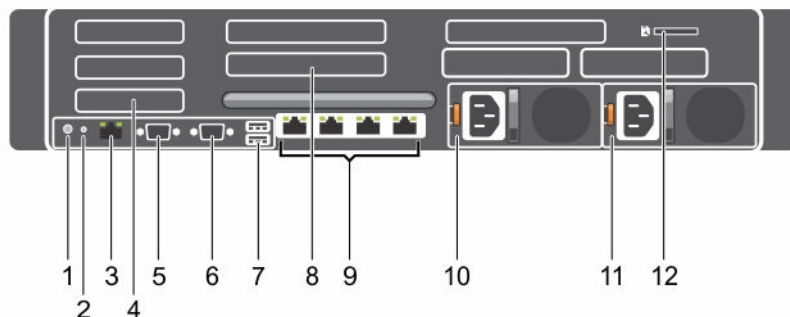
図 4. 背面パネルの機能とインジケータ
