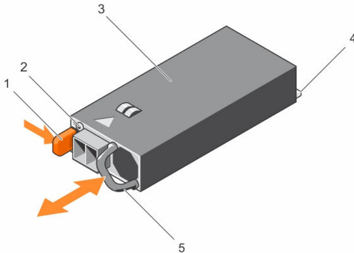
図 43. DC 電源装置の取り外しと取り付け
