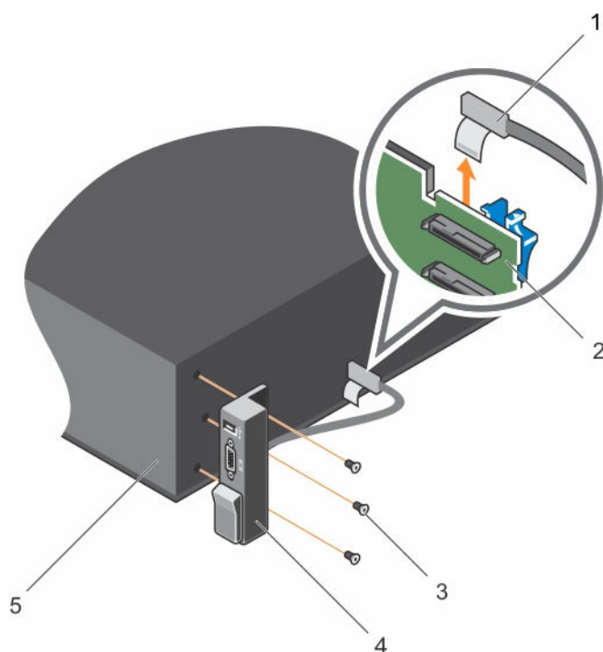
図 53. I/O パネルの取り外しと取り付け
