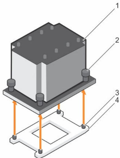
図 18. プロセッサの取り外しと取り付け
