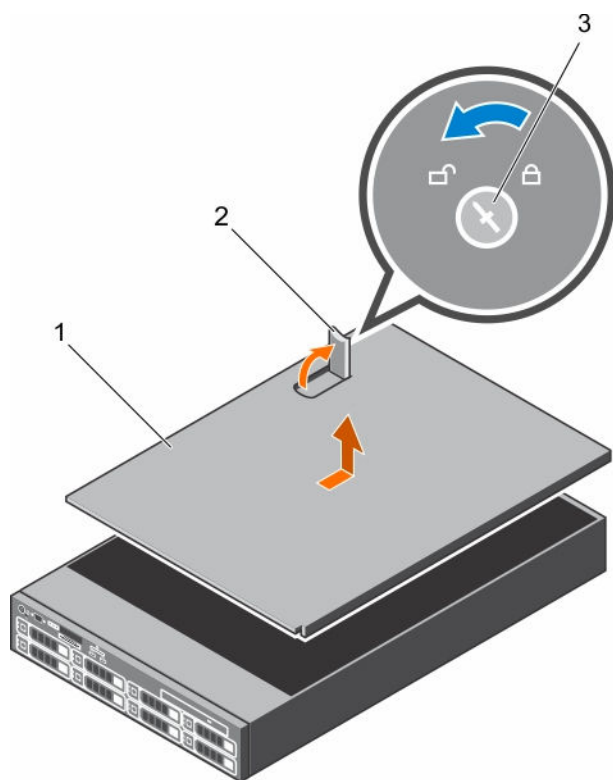
図 9. システムカバーの取り外し
