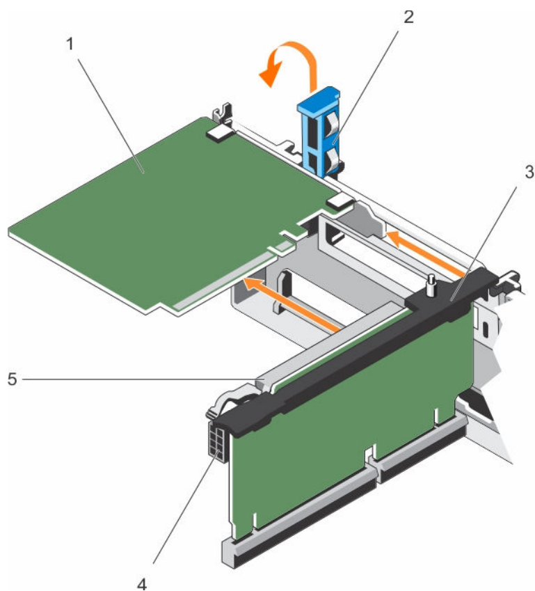
図 28. 拡張カードライザー 2 または 3 からの拡張カードの取り外しと取り付け
