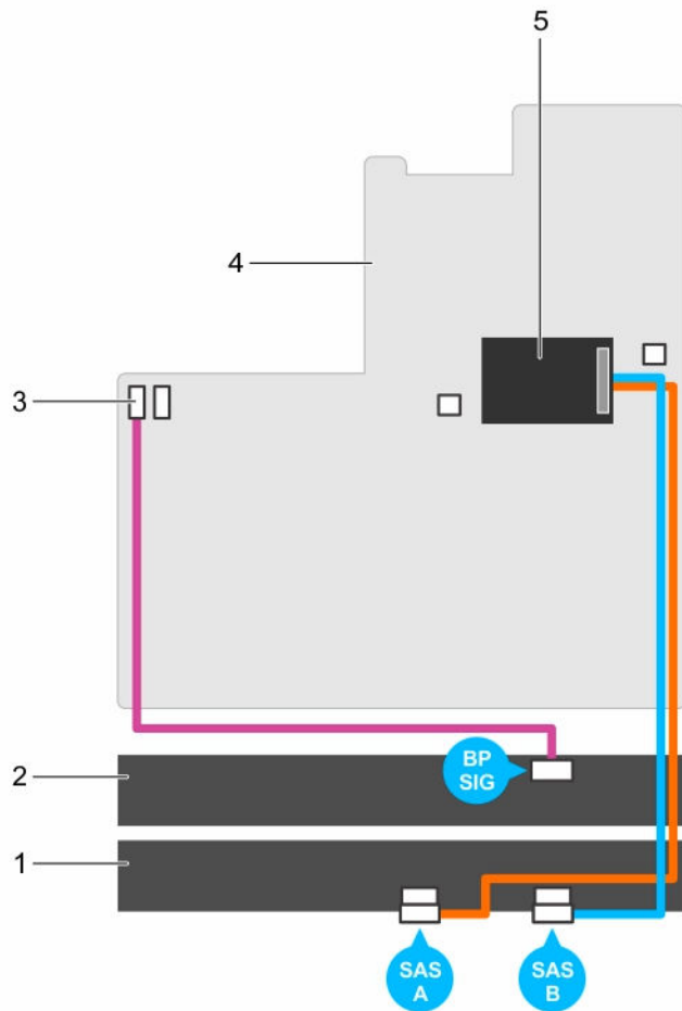
図 50. ケーブル配線図 – 2.5 インチ (x16) SAS/SATA バックプレーン
