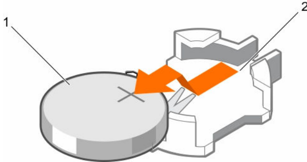
図 40. システムバッテリーの取り外し
