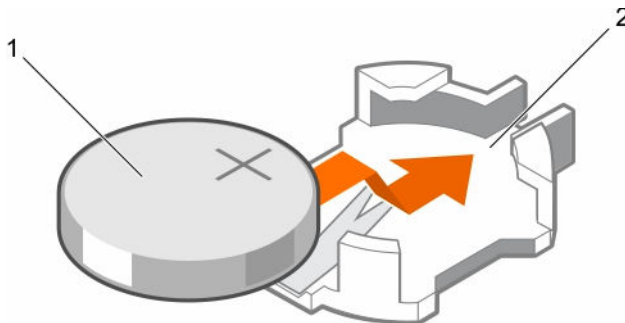
図 41. システムバッテリーの取り付け
