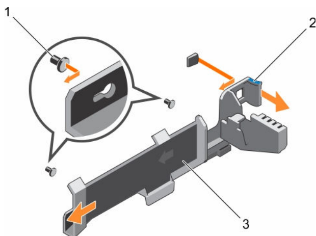
図 26. ケーブル固定ブラケットの取り外しと取り付け
