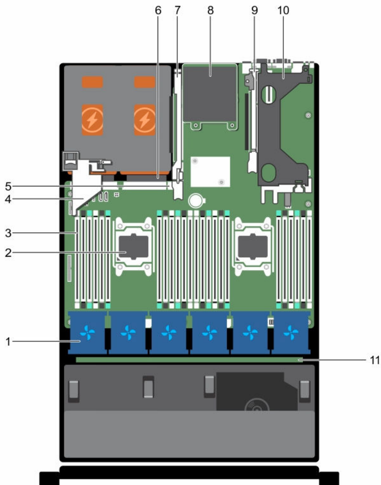
図 10. システム内部 – Dell XC730-16G
