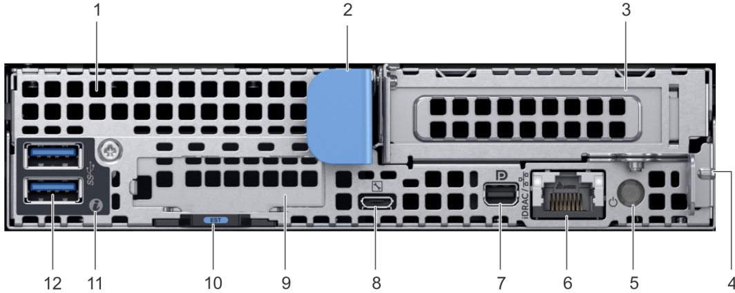
Rakam 1. XC6420 Serisi kızığın arkadan görünümü
