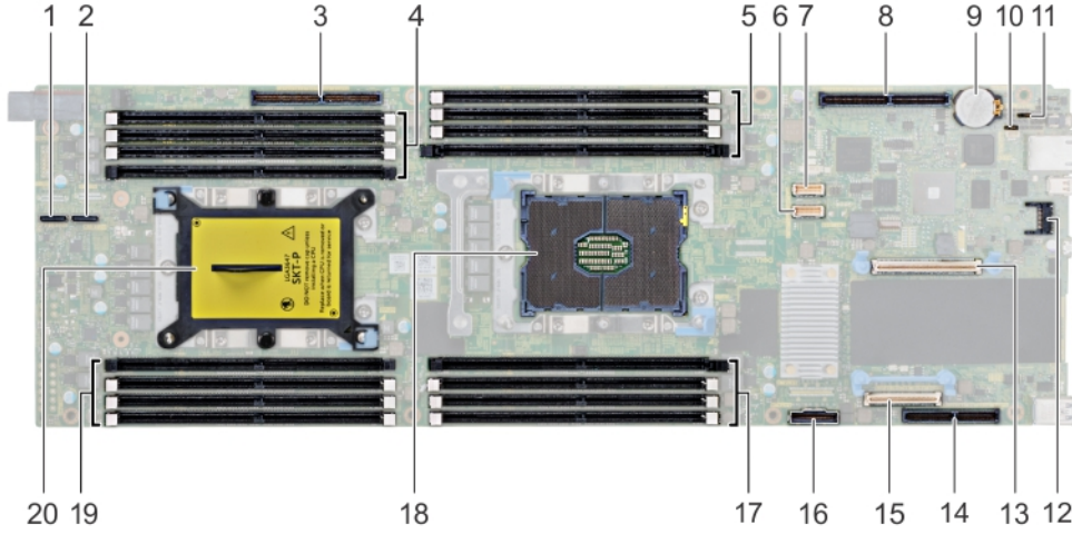
Rakam 41. XC6420 sistem kartı konektörleri
