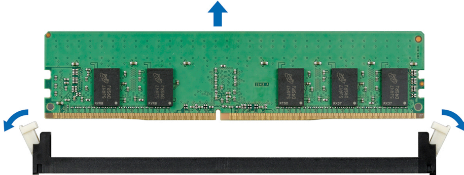
Rakam 16. Bellek modülünü çıkarma
