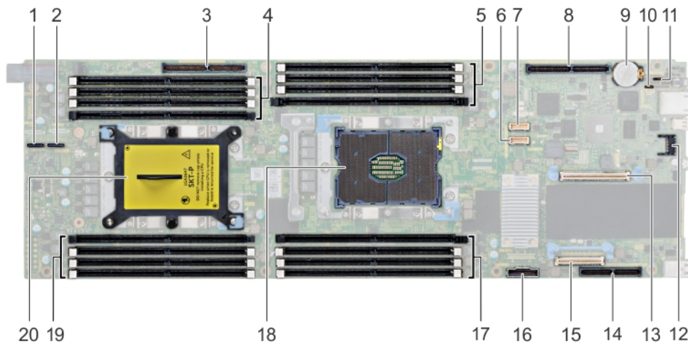
図 41. XC6420 システム基板コネクタ
