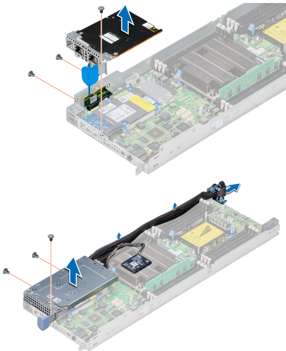
図 32. メザニンカードの取り外し
