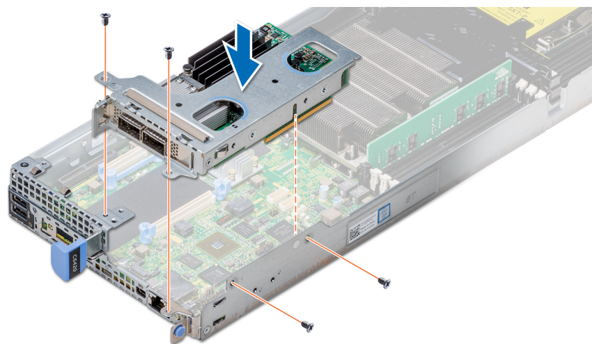
図 21. 拡張カードライザーアセンブリの取り付け
