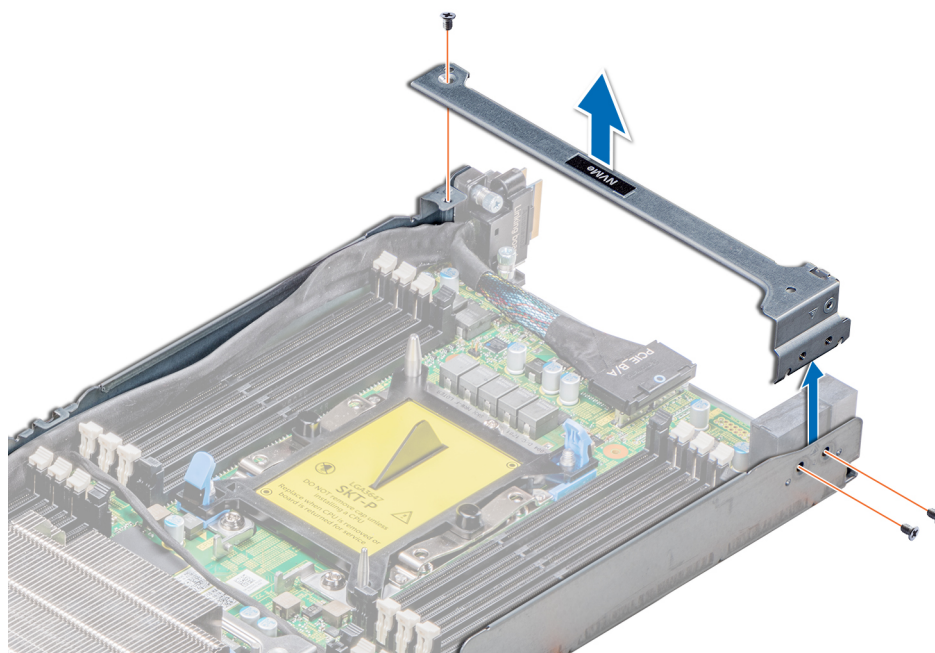
図 18. サポート ブラケットの取り外し
