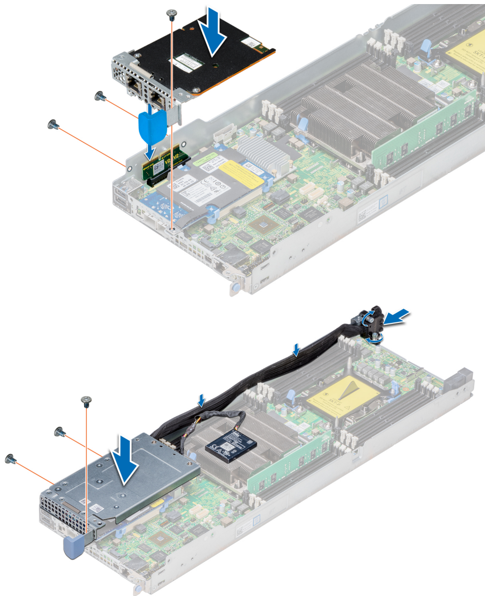
図 33. メザニンカードの取り付け
