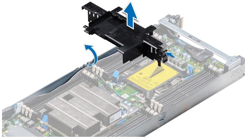
図 13. エアフローカバーの取り外し
