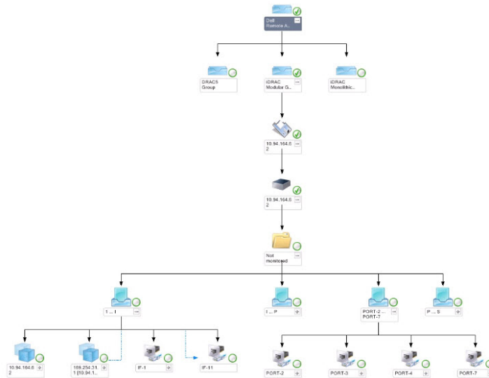
그림 4. 원격 액세스 컨트롤러 그룹 다이어그램
