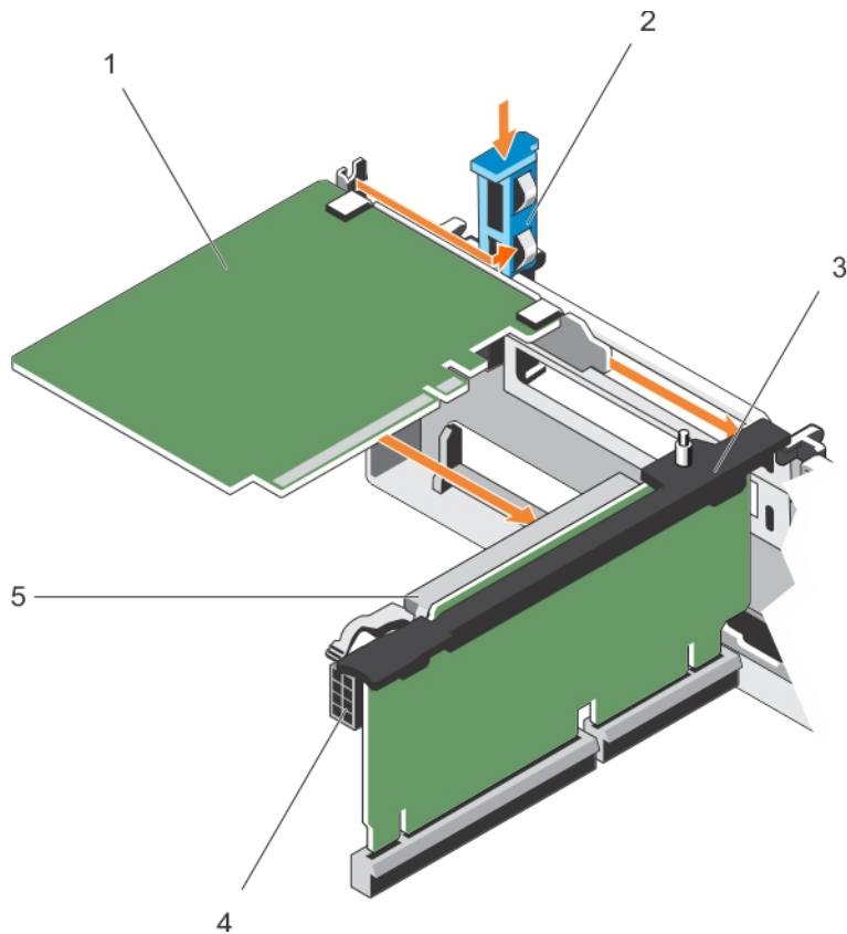
Abbildung 34. Installieren einer Erweiterungskarte im Erweiterungskarten-Riser 2 oder 3
