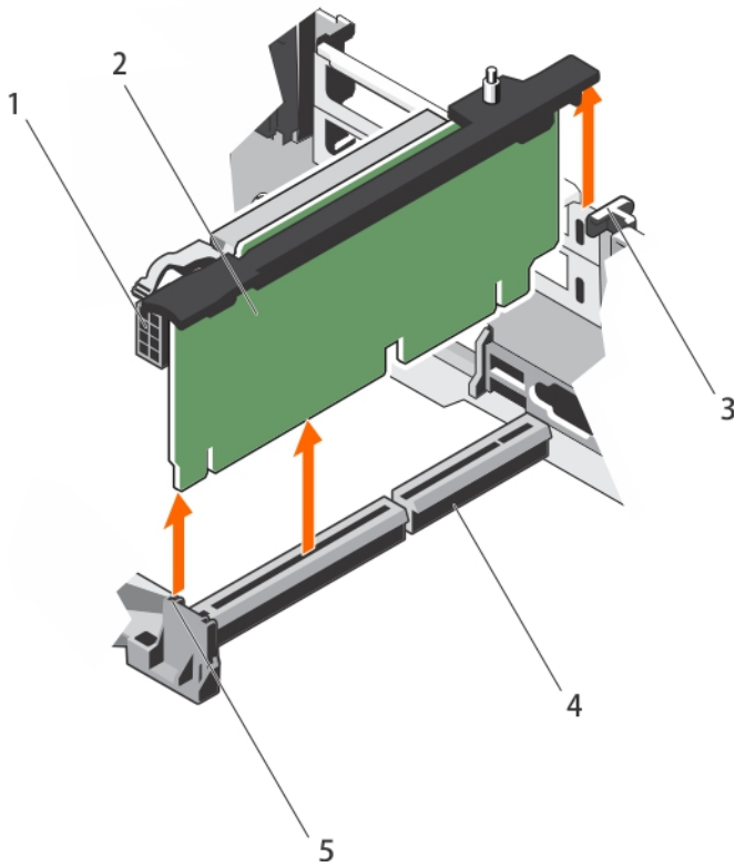
Abbildung 41. Entfernen des Erweiterungskarten-Risers 2
