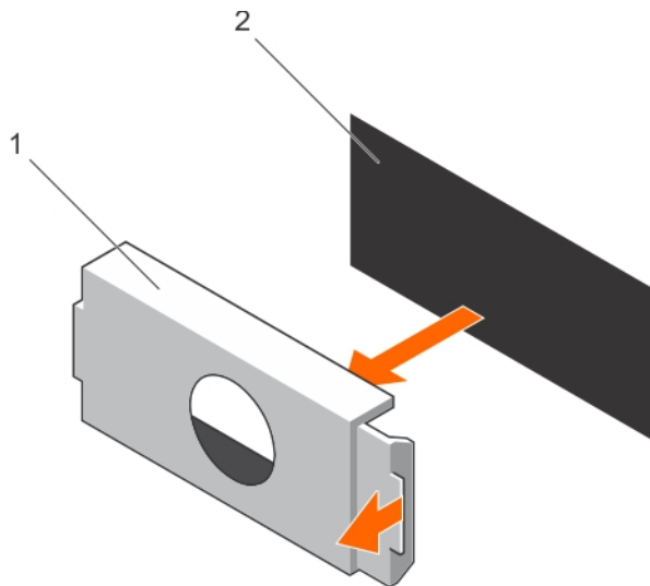
Abbildung 58. Entfernen der Netzteilplatzhalterkarte
