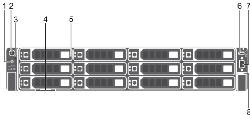
Abbildung 1. Das Dell DR4300e-System - Funktionen und Anzeigen auf der Vorderseite
