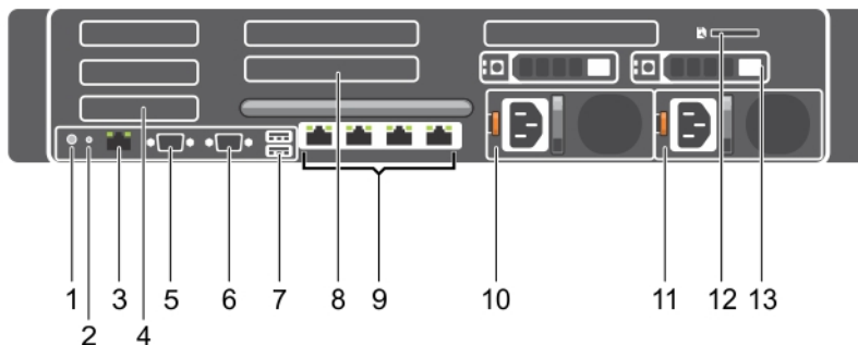
Abbildung 2. Rückseitenmerkmale
