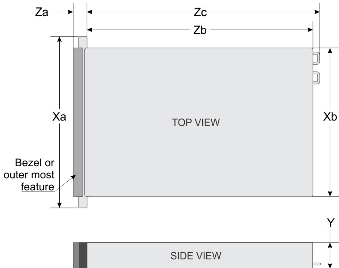
Abbildung 8. Gehäuseabmessungen des Dell DR4300e-Systems
