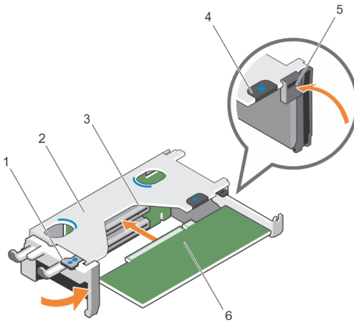
Abbildung 36. Einsetzen einer Erweiterungskarte in den Erweiterungskarten-Riser 1
