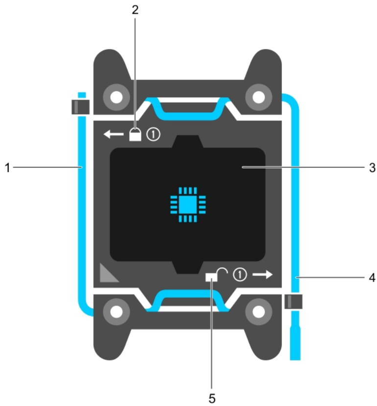
Abbildung 21. Prozessorabdeckung
