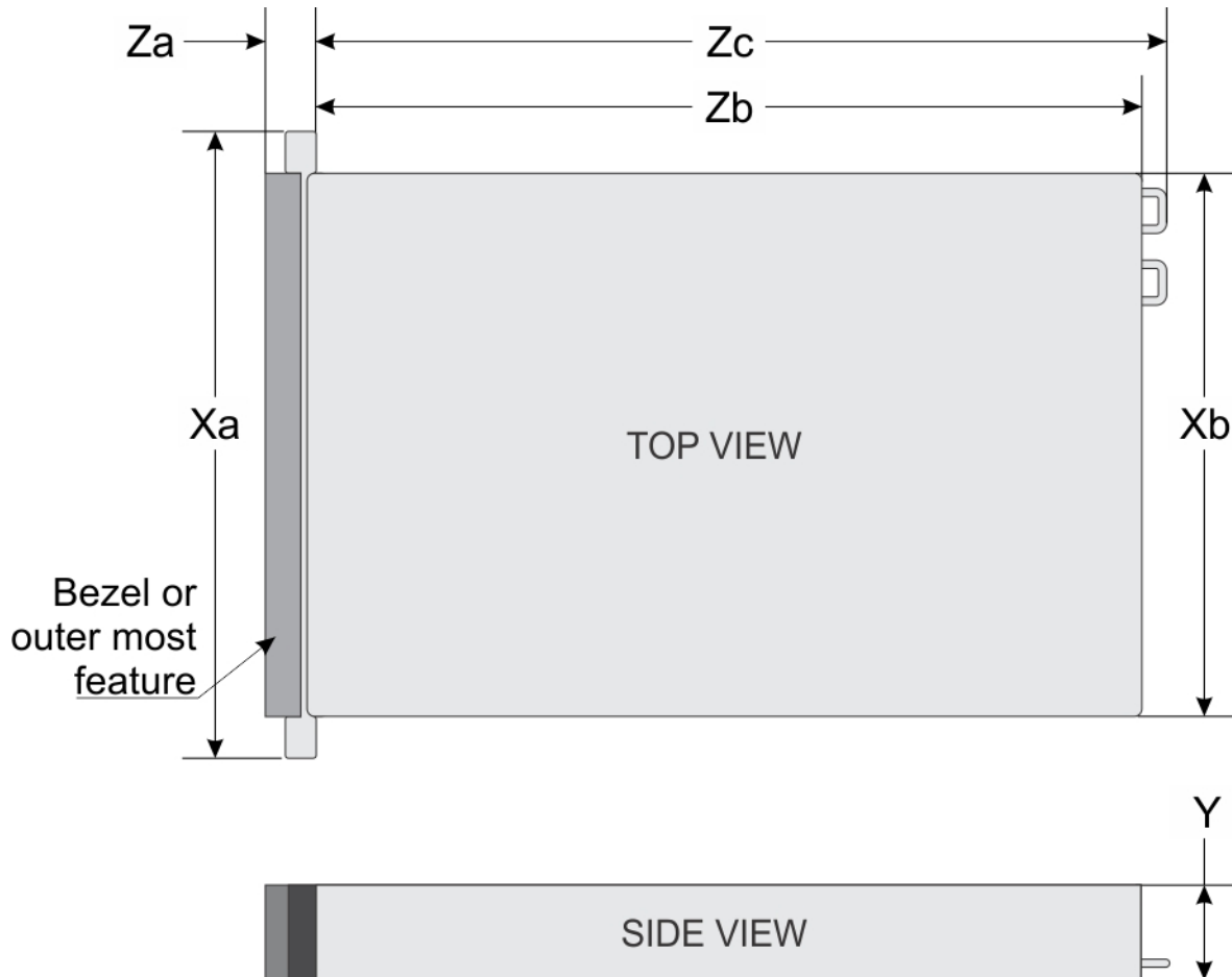
図 7. Dell DR4300 システムのシャーシ寸法
