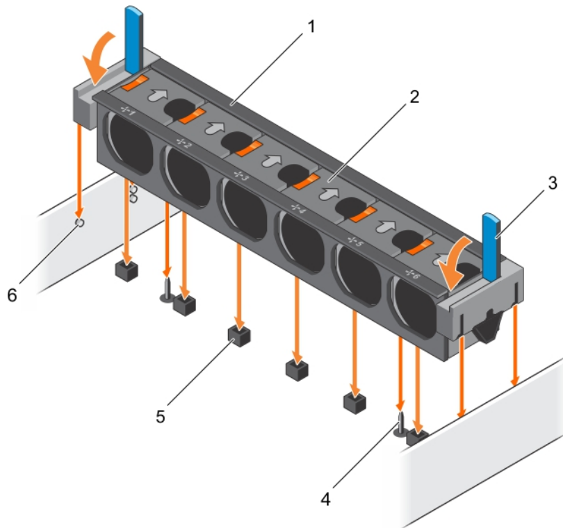
図 15. 冷却ファンアセンブリの取り付け
