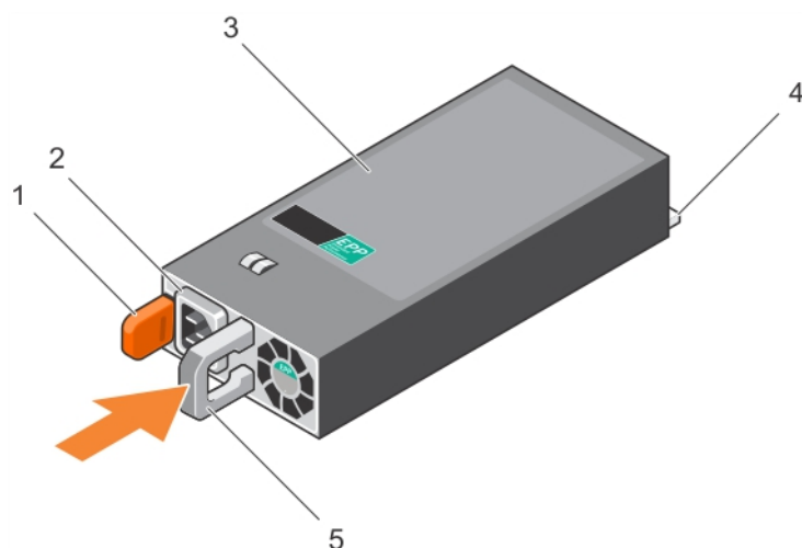
Figure 60. Installation d'un bloc d'alimentation (PSU) CA
