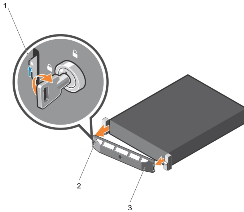
Figure 8. Retrait du cadre avant en option.
