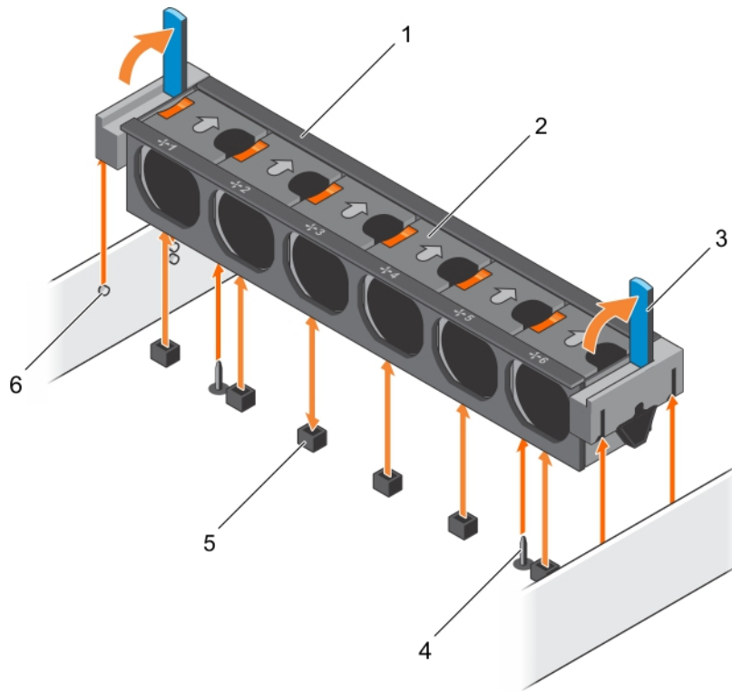
Figure 14. Retrait de l'assemblage de ventilation
