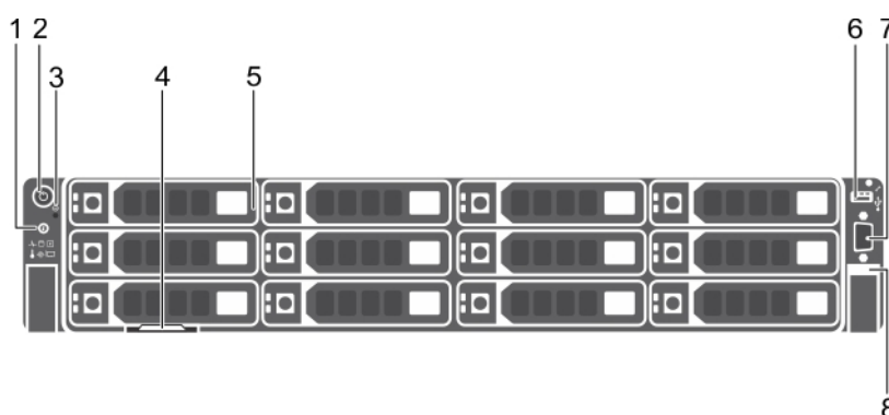
Figure 1. Fonctions et voyants du panneau avant du système Dell DR4300
