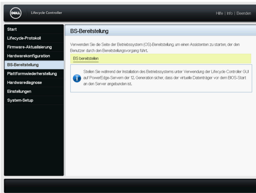
Abbildung 9. Seite BS-Bereitstellung
