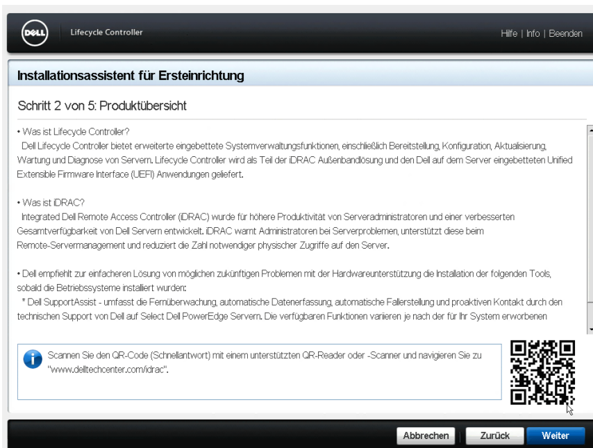
Abbildung 4. Produktübersicht-Seite
