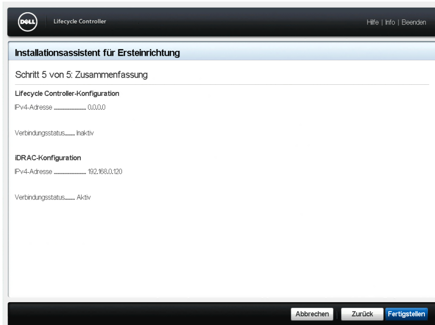
Abbildung 7. Zusammenfassingsseite
