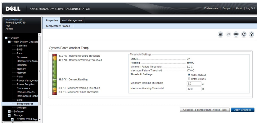
Abbildung 3. Messanzeige
