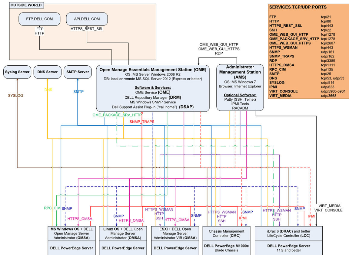
図 12. ネットワーク接続
