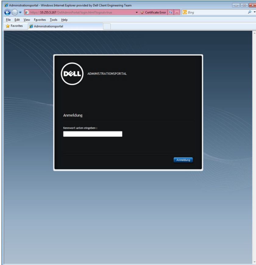
Abbildung 3. Verwaltungskonsole
