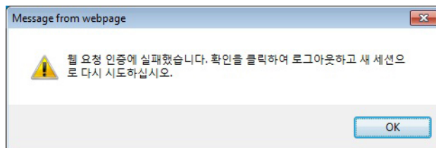
그림 1. 오류 메시지
