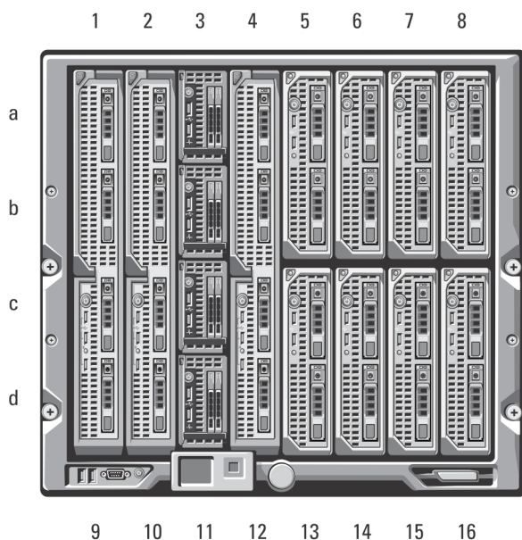
图 4: 刀片编号 - 混合的全高、半高和四分之一高度刀片
