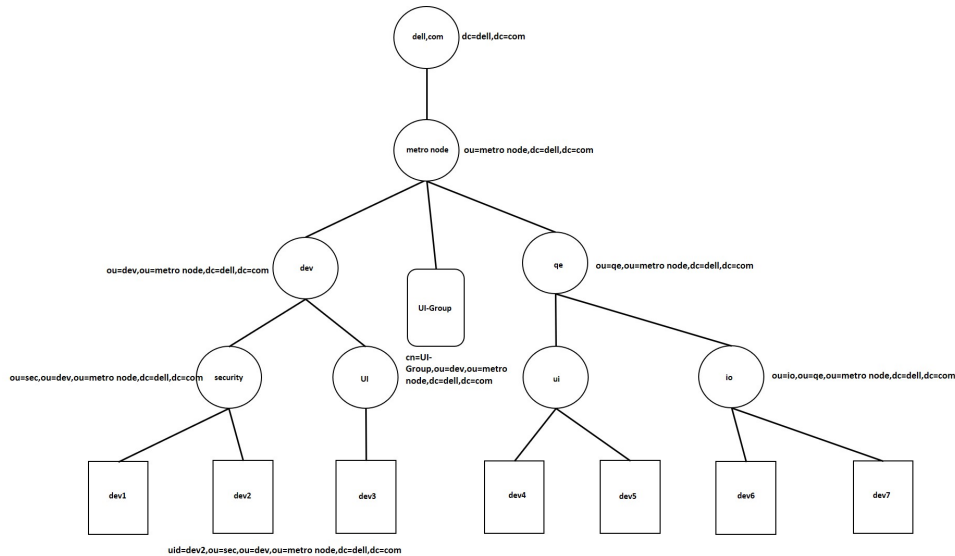
Figure 4. Structure de répertoire LDAP
