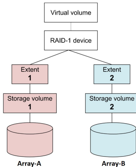
Figure 3. Géométries courantes : RAID 1 à deux branches
