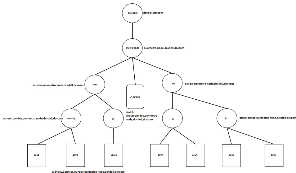
Ilustración 4. Estructura de directorios LDAP
