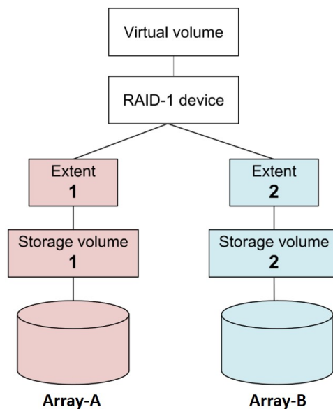
Ilustración 3. Geometrías comunes, RAID 1 de dos secciones
