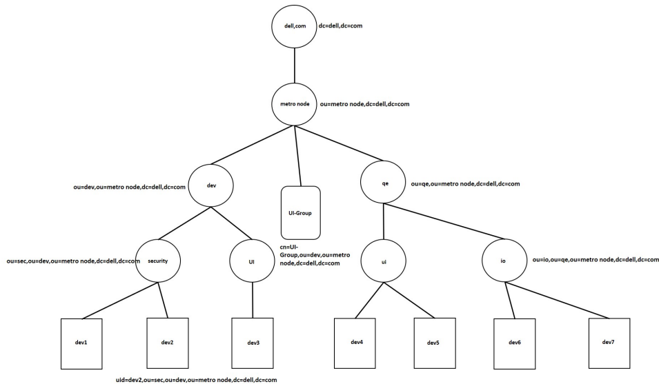
Abbildung 4. LDAP-Verzeichnisstruktur
