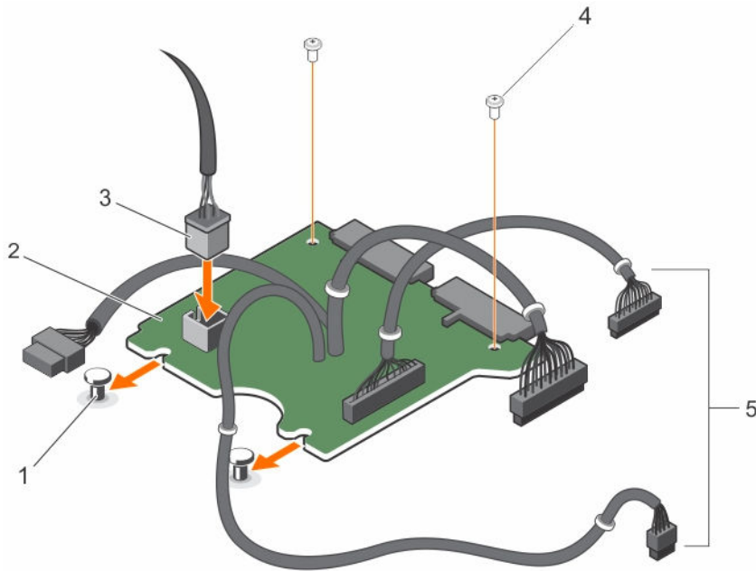
Abbildung 72. Einbauen des PIB
