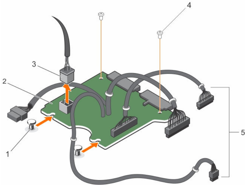
Abbildung 71. Entfernen der PIB
