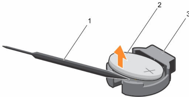
Abbildung 55. Entfernen der Systembatterie
