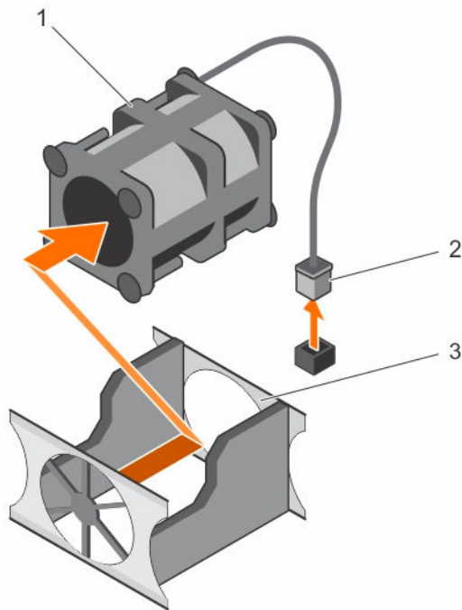
Abbildung 33. Entfernen eines Kühlungsüfters
