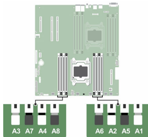
Abbildung 18. Positionen der Speichersocket
