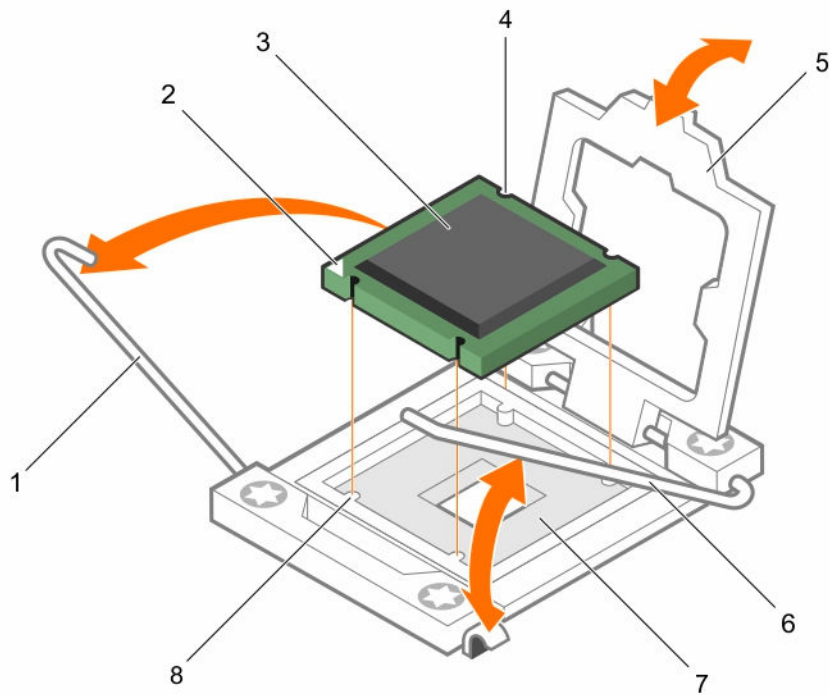
Abbildung 44. Entfernen eines Prozessors
