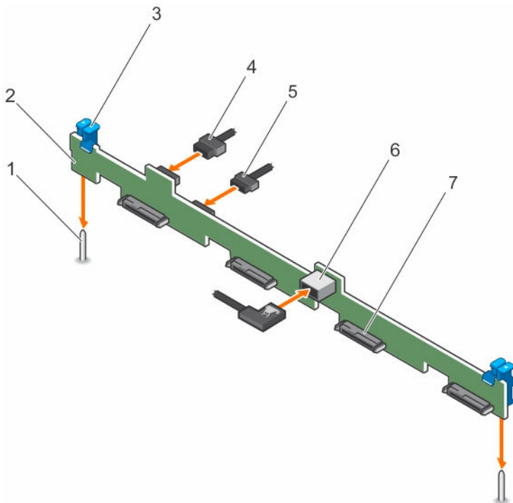
Abbildung 61. Installieren der Rückwandplatine für vier 3,5-Zoll-SAS/SATA-Festplatten
