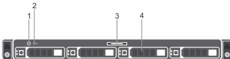
Abbildung 2. Funktionsmerkmale auf der Frontblende eines 4 x 3,5- Zoll Festplattengehäuses
