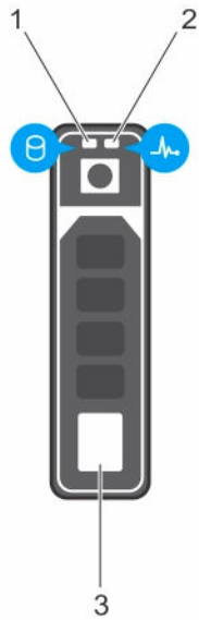
Abbildung 6. Laufwerksanzeigen
