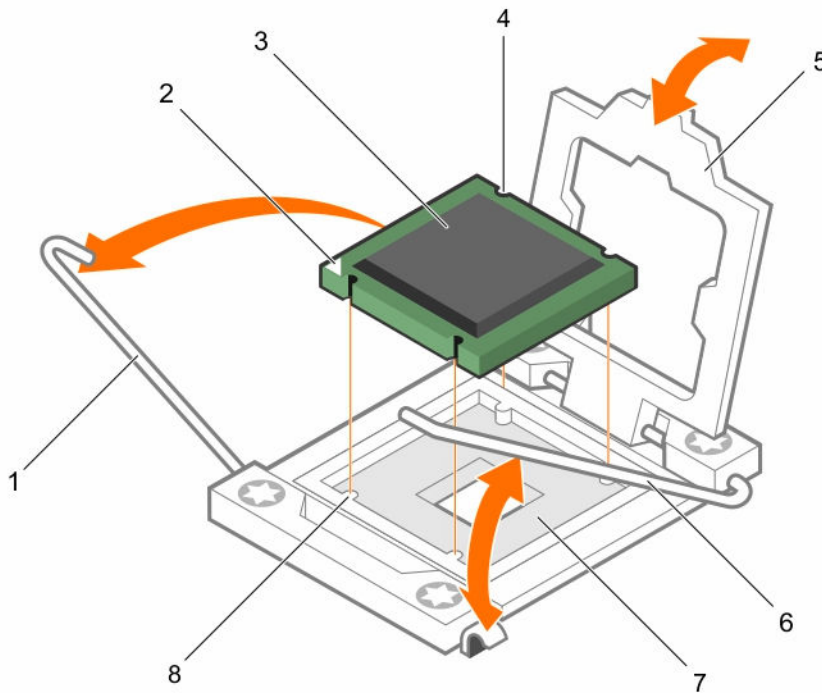
Abbildung 45. Einsetzen eines Prozessors
