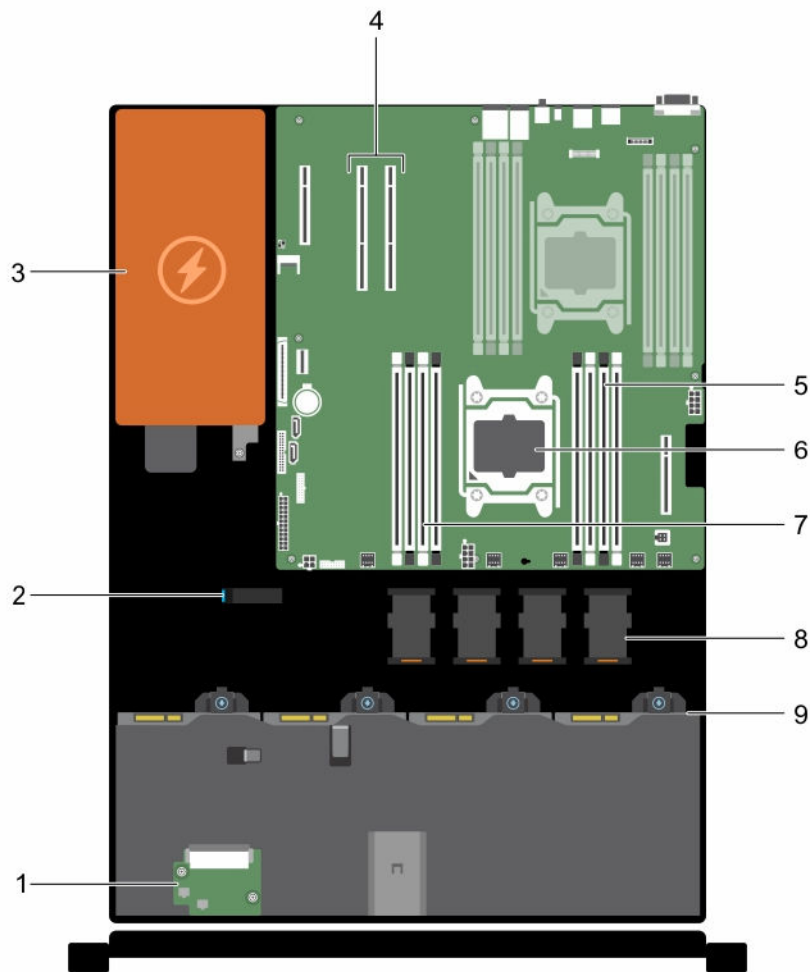
Abbildung 15. Das Systeminnere - mit nicht-redundanter PSU
