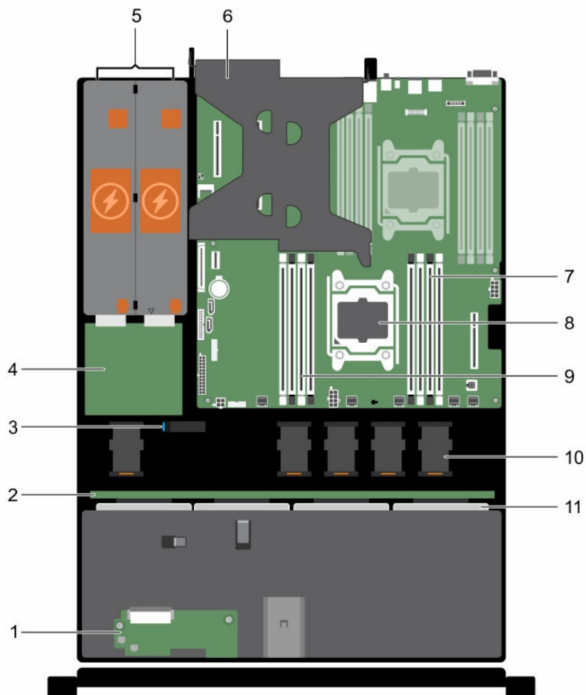
Abbildung 14. Das Systeminnere – mit einer nicht redundanten Netzteilereinheit (PSU)
